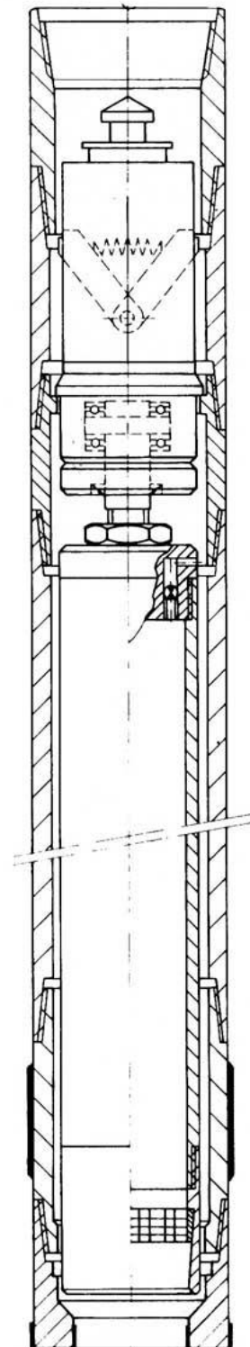
Seilkernrohr
