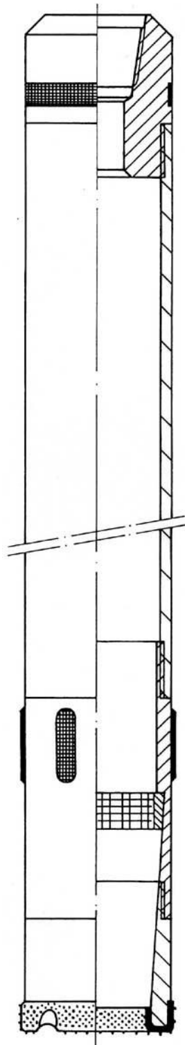
Einfachkernrohr
