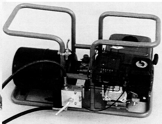
Hydraulikaggregat Typ 1112
