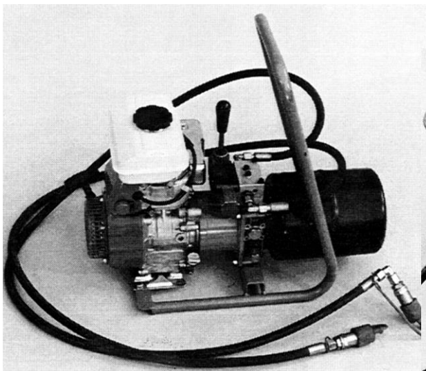
Hydraulikaggregat Typ 35
