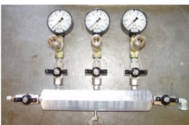
Druckluftverteiler
