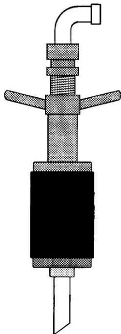
Mechanischer Packer mit Stopfbüchse für Injektionslanze
