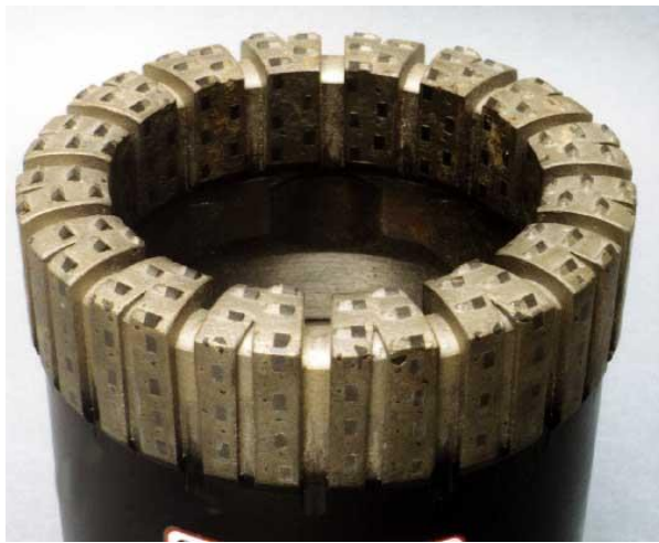
Synset-Diamantbohrkrone mit 16 Spülungswegen
