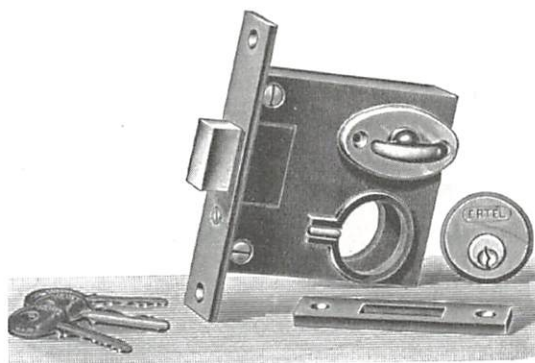
Auch Einsteckschlösser für schwere Türen und Tore bauten die Ertel-Werke München Anfang der 1920er-Jahre
