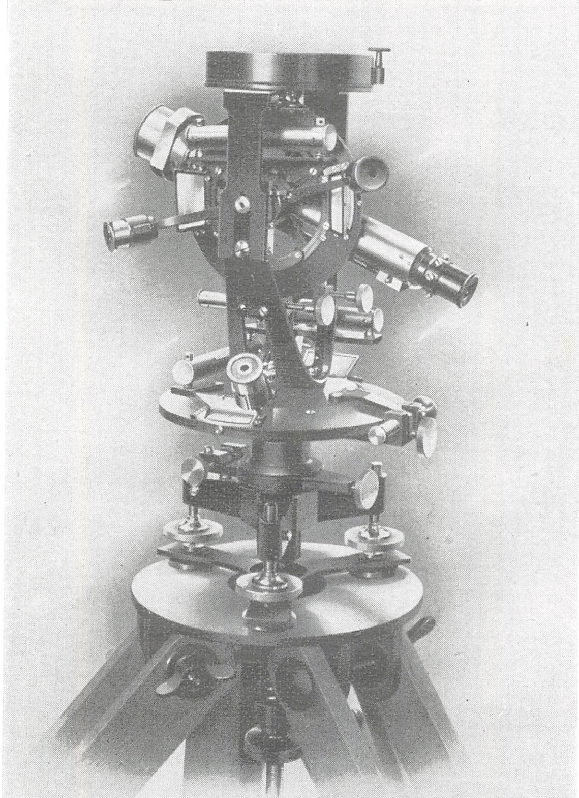
Ertel Normal Repetitions- Theodolit (um 1920)
