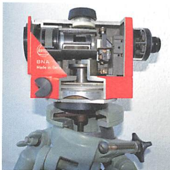
BNA Schaumodell, aufgeschnitten
