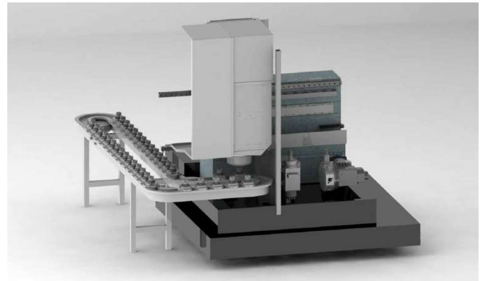
Pick-up-Lösung seitlich
