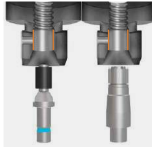
VORSCHLEIFEN / HONEN
