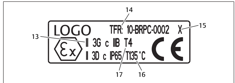
Abb. 3: ATEX-Schild für Zone 3G 3D
