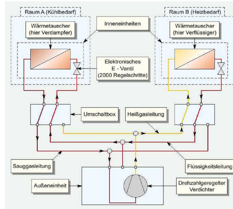
Schema des Wärmepumpensystems zur internen Wärmeverschiebung (VRV-Invertersystem)
