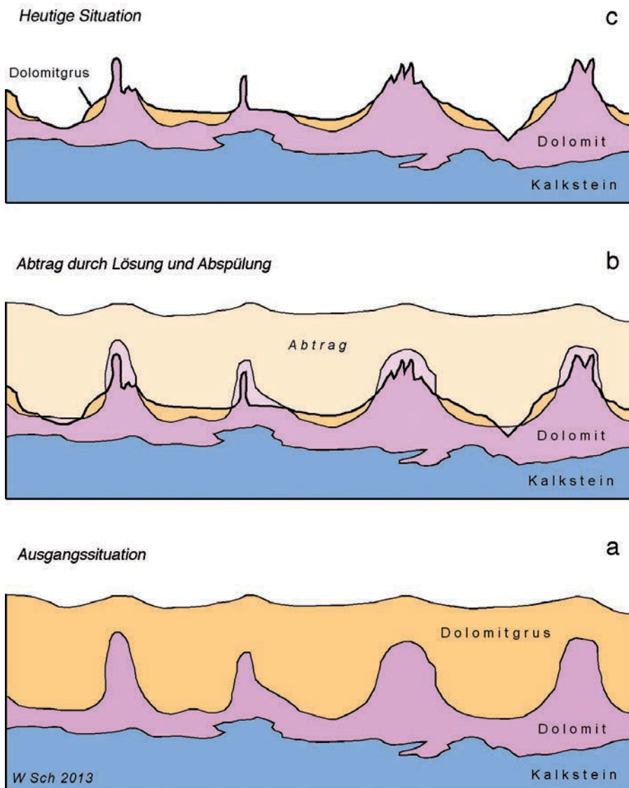
Bild 2 Prinzipielles Schema der Entstehung der Dolomitturlandschaft der Nördlichen Frankenalb.
