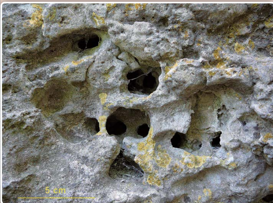
Bild 9 Kleinlöcher im Dolomit am Breitenberg bei Gößweinstein.
