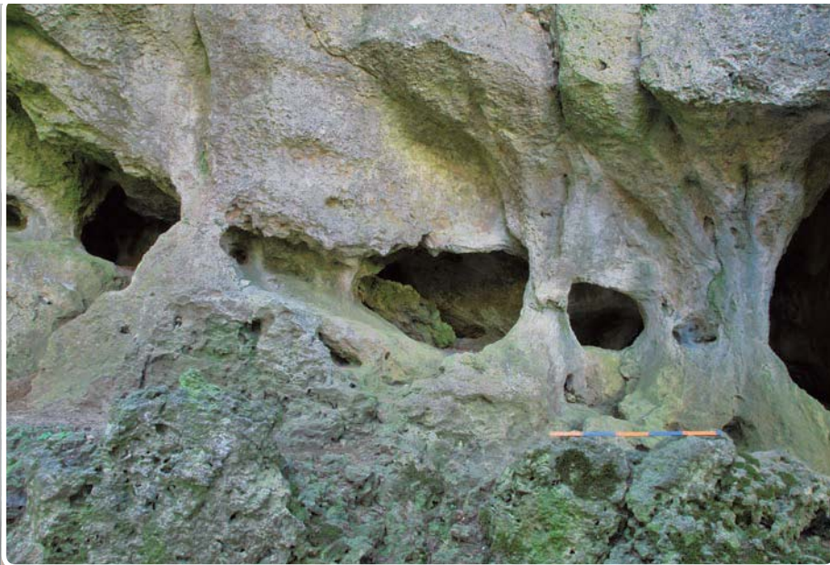
Bild 8 Galerieartige Fenster-Höhle im Dolomit des Wasserstein-Felsmassivs nördlich Betzenstein. Maßstab 50 cm. Hinter den Fensterstegen als Reste einer Wandkruste breitet sich der Höhlenraum durchgehend aus.
