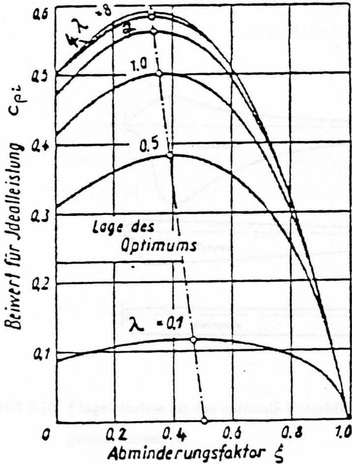
Bild 2.8: Idealer Leistungsbeiwert c_{pi} als Funktion des Abminderungsfaktors \xi mit der Schnellaufzahl \lambda als Parameter [11]
