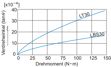
Abb.9 Vergleich zwischen LBS und LT hinsichtlich Spielfreiheit
