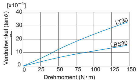
Abb.10 Vergleich zwischen LBS und LT hinsichtlich CL-Spiel
