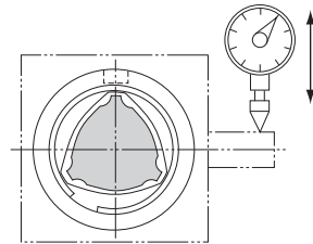
Abb.7 Messung des Spiels in Drehrichtung
