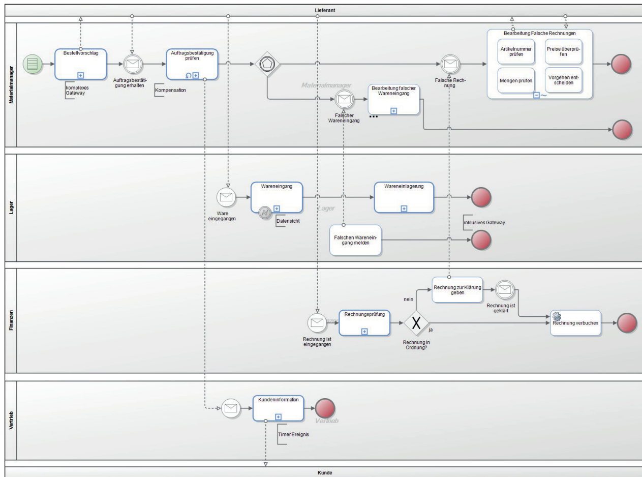
BPMN-Diagramm mit aufgeklapptem Ad-hoc-Teilprozess
