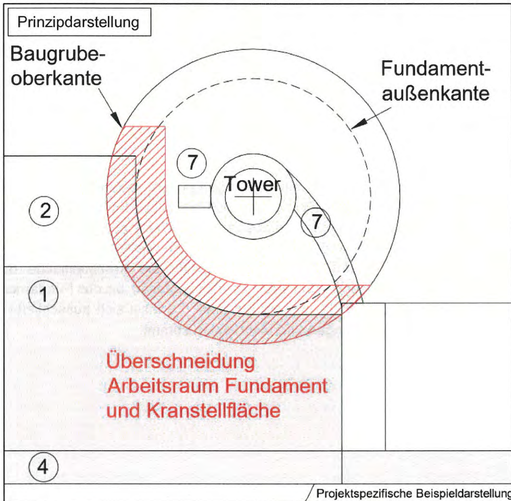
Abbildung 2: Überschneidung Arbeitsraum Fundament und Kranstellfläche
