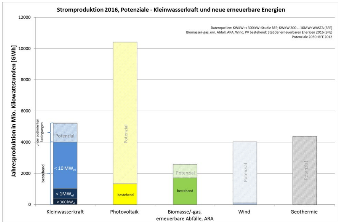
Abb. 18: Jahresproduktion im Vergleich verschiedener erneuerbarer Technologien
