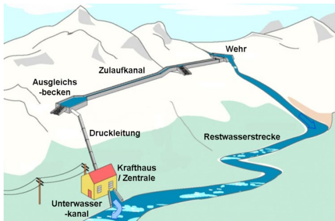
Abb. 16: Schematische Darstellung eines Ausleitkraftwerks
