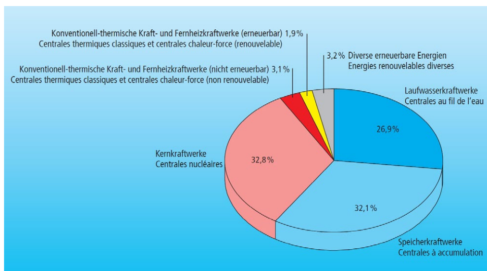
Abb. 12: Produktionsmix der Schweiz, gemäss der Schweizerischen Elektrizitätsstatistik 2016 des BFE
