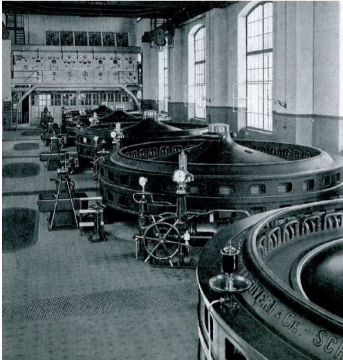
Abb. 13: Hagneckwerk, Maschinensaal (1914) [23]
