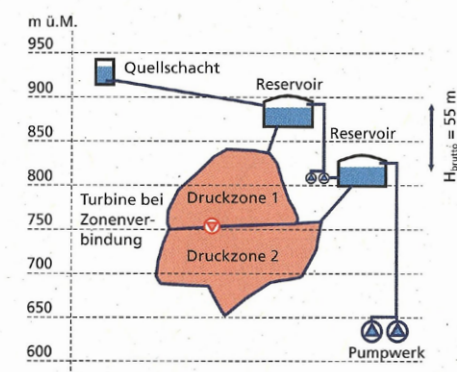
Abbildung 3-3 Stromerzeugung am Druckbrecher zwischen zwei Zonen, [24]
