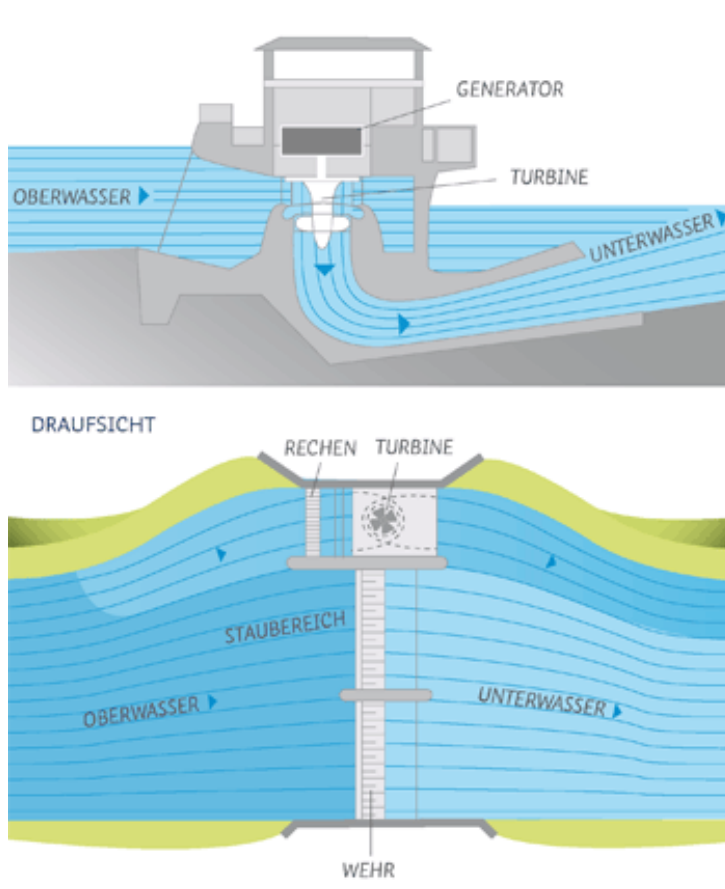
Abbildung 2-3 Schema Durchlaufkraftwerk, [4]
