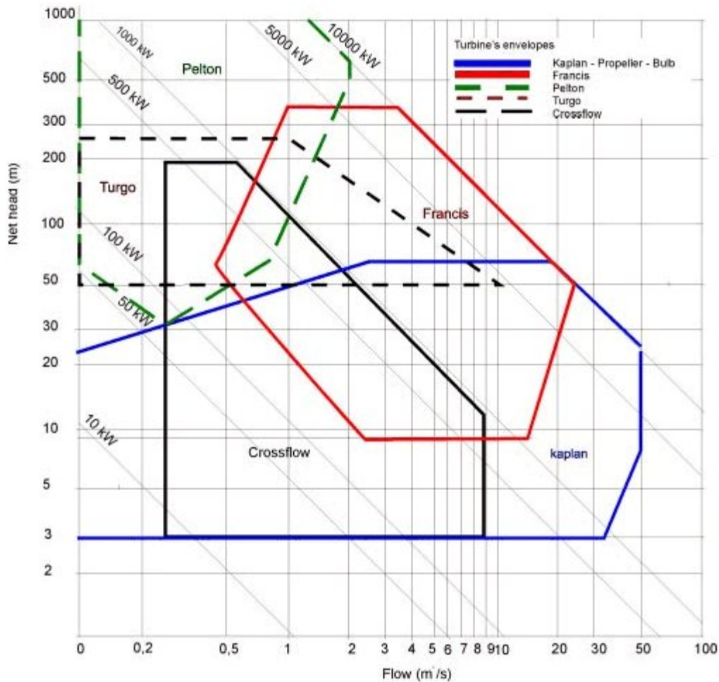
Abbildung 2-17 Anwendungsbereich von Turbinen [12]
