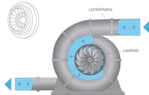
Francis-Turbine
