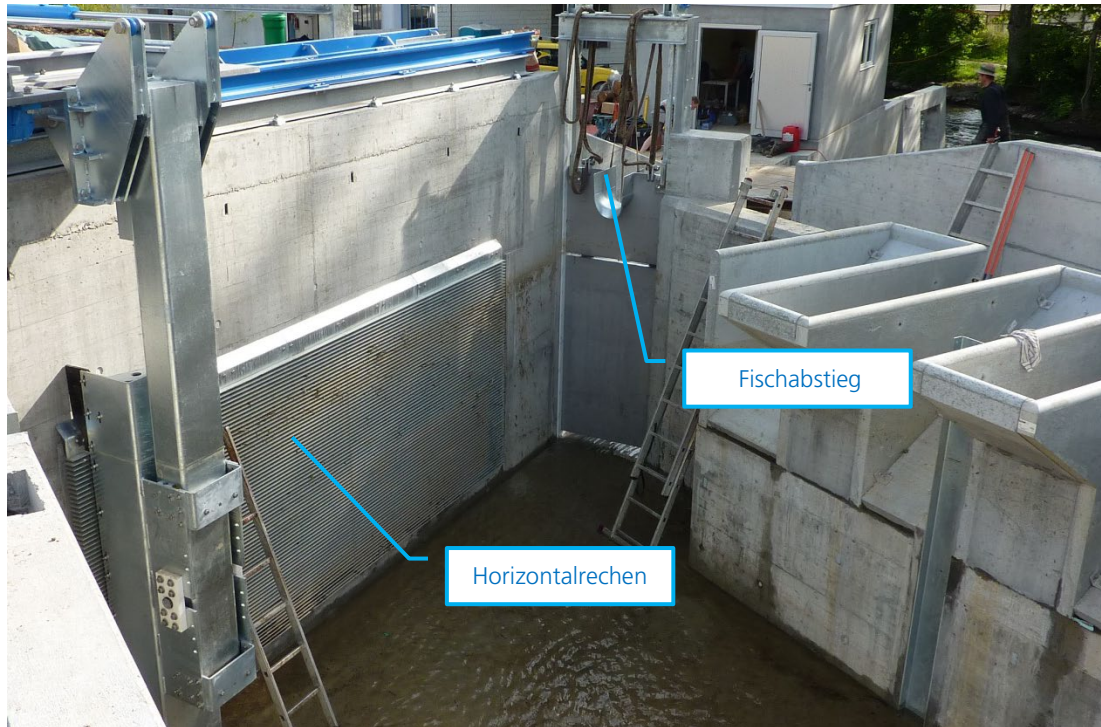
Abbildung 6-2 Horizontalrechen und Fischbypass am KW Hämmerli
