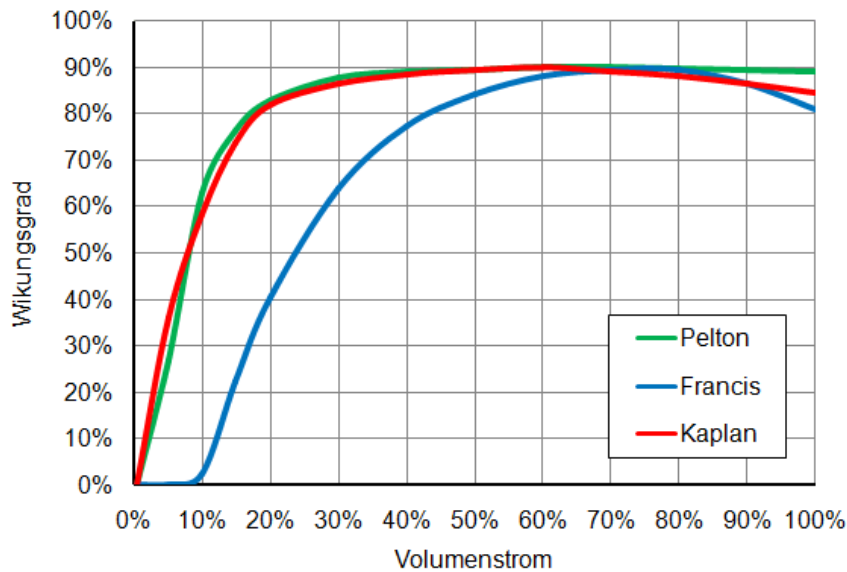
Abbildung 2-18 Wirkungsgrad in Funktion des Volumenstroms. (Normiert auf ein Maximum von 90%). [13]
