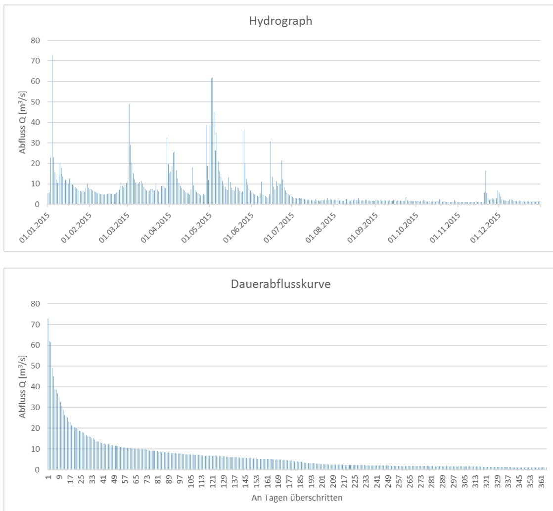
Abbildung 4-5 Hydrograph und Dauerabflusskurve für die Töss in Neftenbach 2015, [33]
