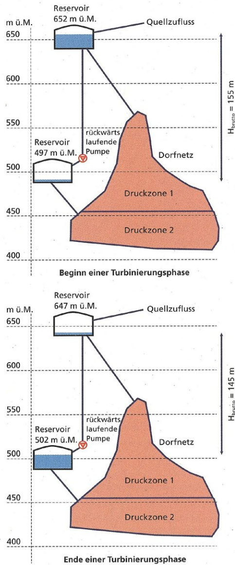
Abbildung 3-1 Integration eines Trinkwasserkraftwerks in die Verbindungsleitung zweier Reservoir, [24]
