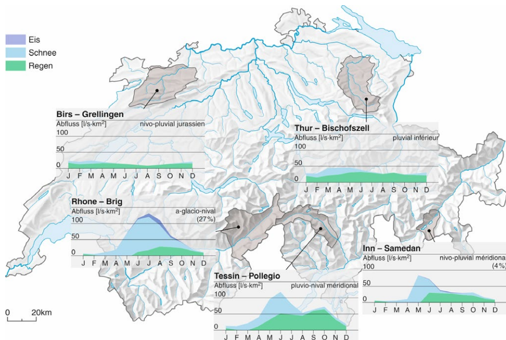
Abbildung 4-6 Abflussregimes für fünf repräsentative Einzugsgebiete aus verschiedenen Regionen der Schweiz für die Periode 1984 bis 2005, [34]
