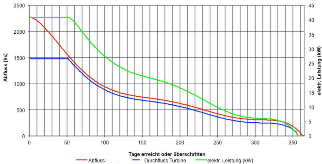
Abbildung 4-7 Leistungsplan für ein Kraftwerk
