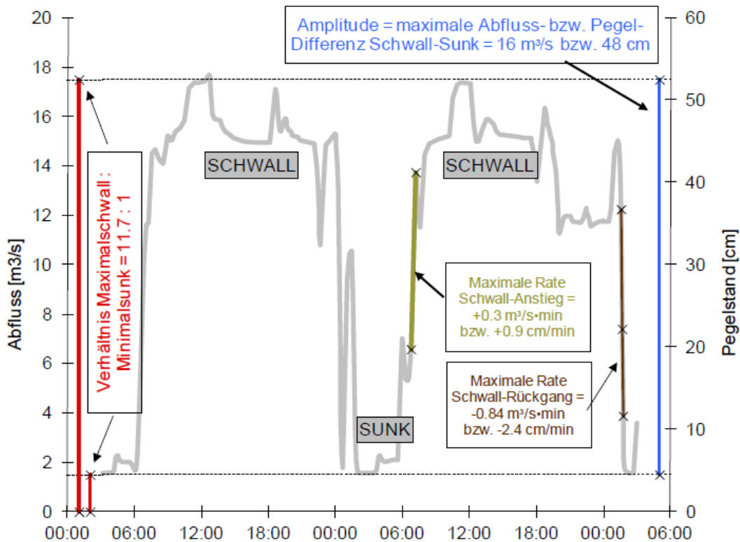
Abbildung 6-3 Wichtige Kennwerte des Schwallbetriebes, dargestellt anhand der Abfluss- bzw. Pegelganglinie, [65]
