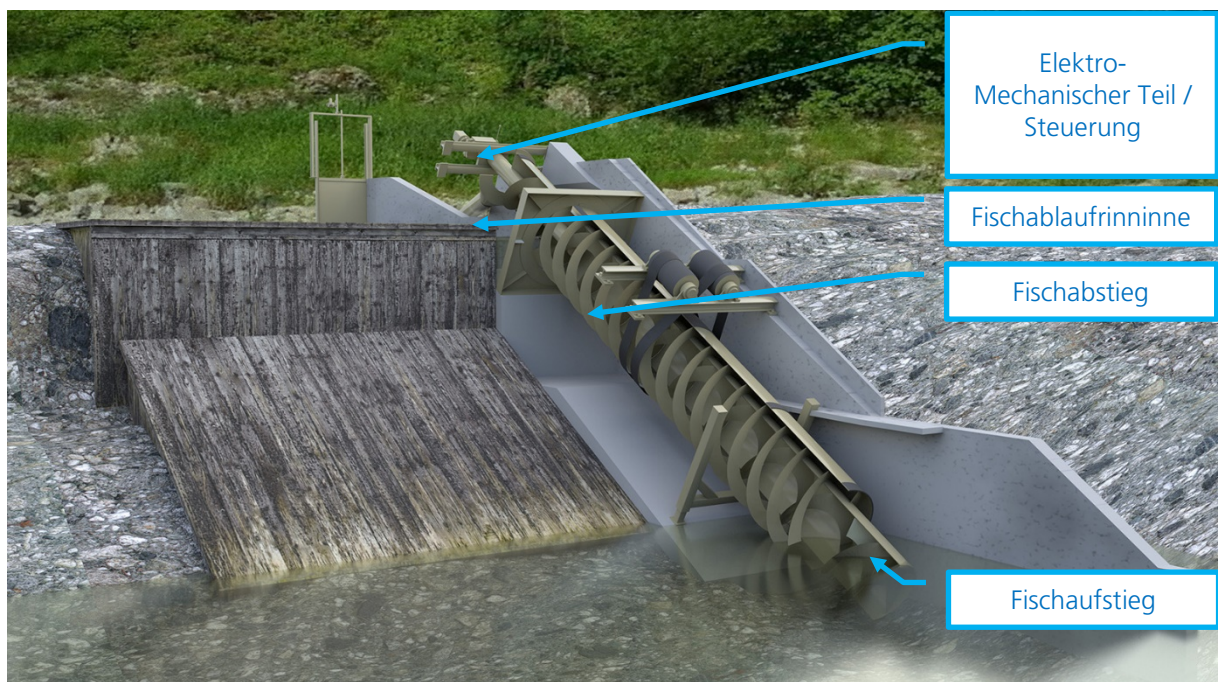
Abbildung 2-20 Prinzipschema eines Drehrohr-Doppelwasserkraftschnecke, [16]
