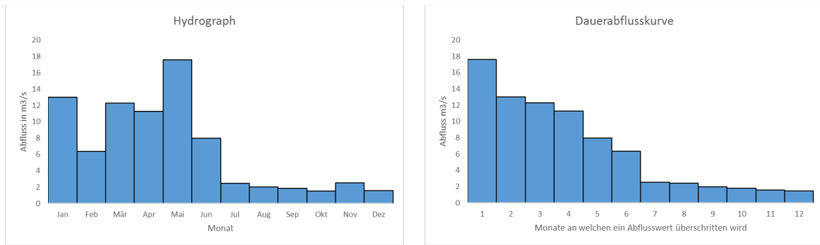
Abbildung 4-4 Hydrograph und Dauerabflusskurve – vereinfacht aus Monatsmittelwerten abgeleitet (normalerweise werden Tagesmittelwerte verwendet)
