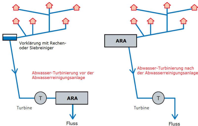
Abbildung 3-4 Schema zur Nutzung von Abwässern zur Stromerzeugung, [23]
