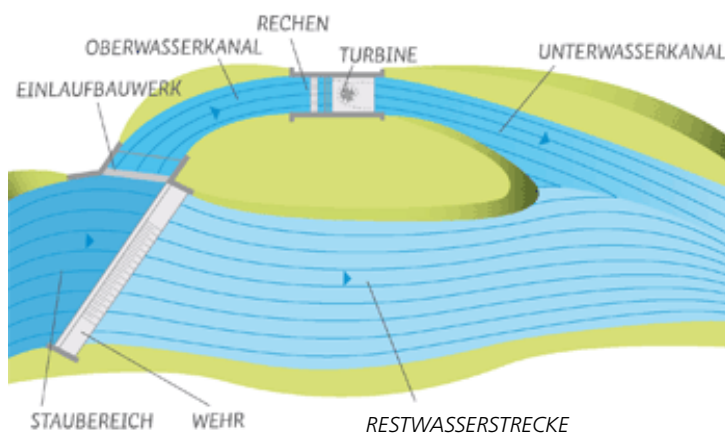
Abbildung 2-2 Schema Ausleitkraftwerk, [4]
