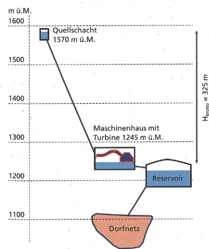
Abbildung 3-2 Nutzung des Quellwasserzulaufs zur Energiegewinnung, [24]
