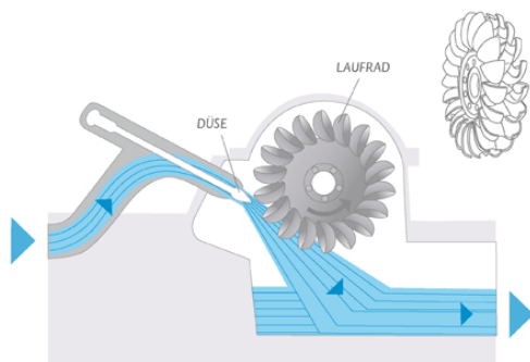
Abbildung 2-16 Die gebräuchlichsten Turbinentypen, [4]
