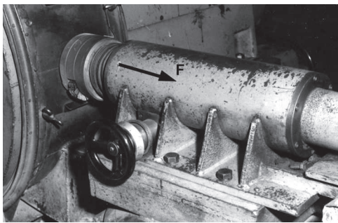
Bild 3.66 Abrichteinrichtung für eine Sonderschleifmaschine
