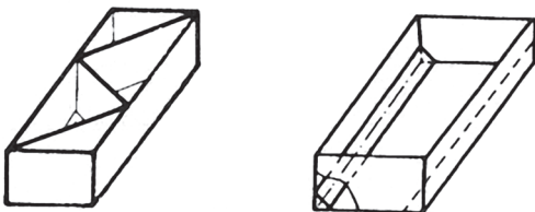
Bild 3.71 Aussteifung offener Kästen für Torsion Links - Dreieckverrippung Rechts - Eckaussteifung
