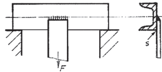
Bild 3.69 Biegeträger mit Verformungsbehinderung durch Zugstababschluss
