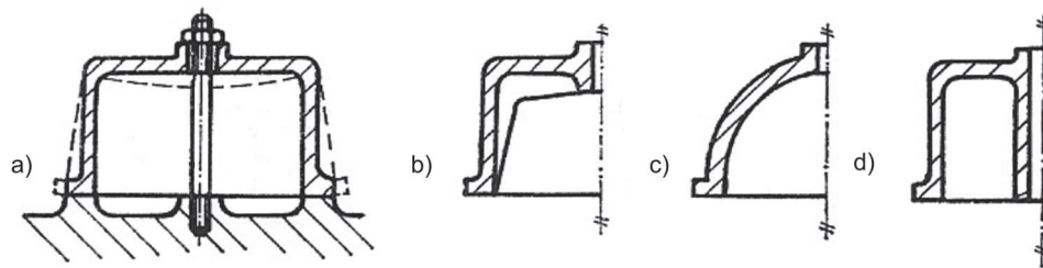
Bild 3.64 Haubenbefestigung [29]
