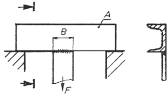
Bild 3.69 Biegeträger mit Verformungsbehinderung durch Zugstababschluss
