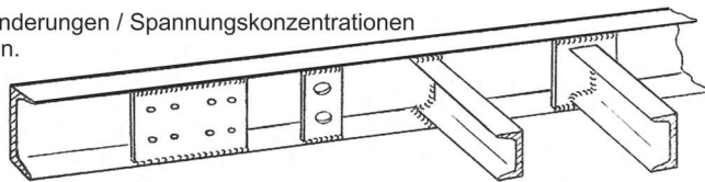
Bild 3.69 Biegeträger mit Verformungsbehinderung durch Zugstababschluss
