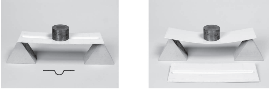
Bild 3.76 Demonstrationsmodelle für Blechversteifungen [45]
