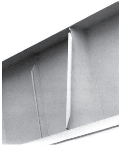
Bild 3.73 Blechversteifung mit Abkantung
