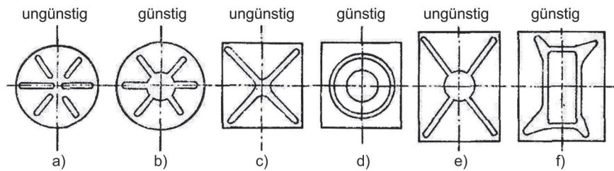
Bild 3.79 Sickenbilder [30]
