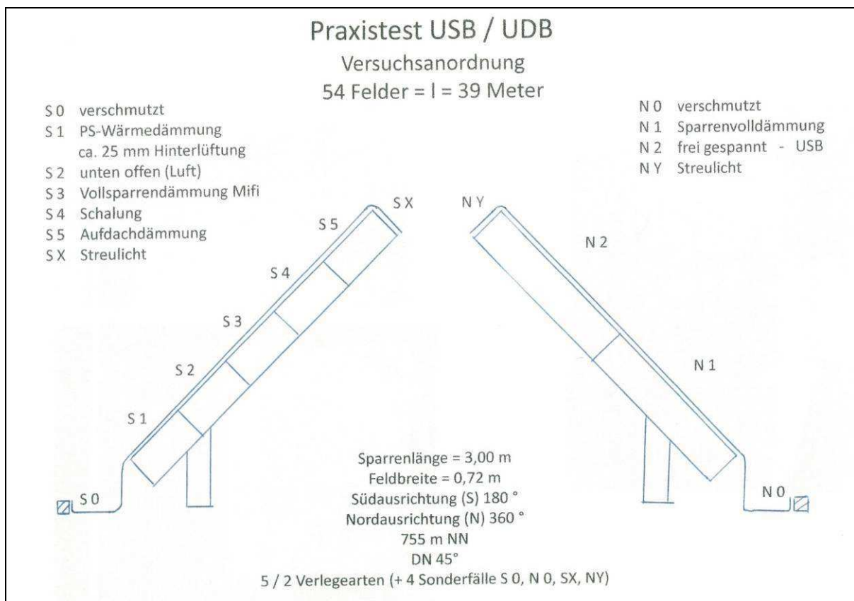
Abb. 26: Schnitt durch die Versuchsanlage mit Feldeinteilungen durch unterschiedliche Einbausituationen.
