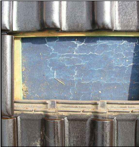
Abb. 33: Craqueléartige Risse der oberen Beschichtung
