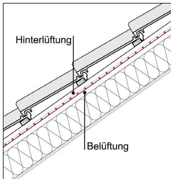
Abb. 10: Belüftete Dachkonstruktion mit Luftspalt oberhalb der Dämmung
