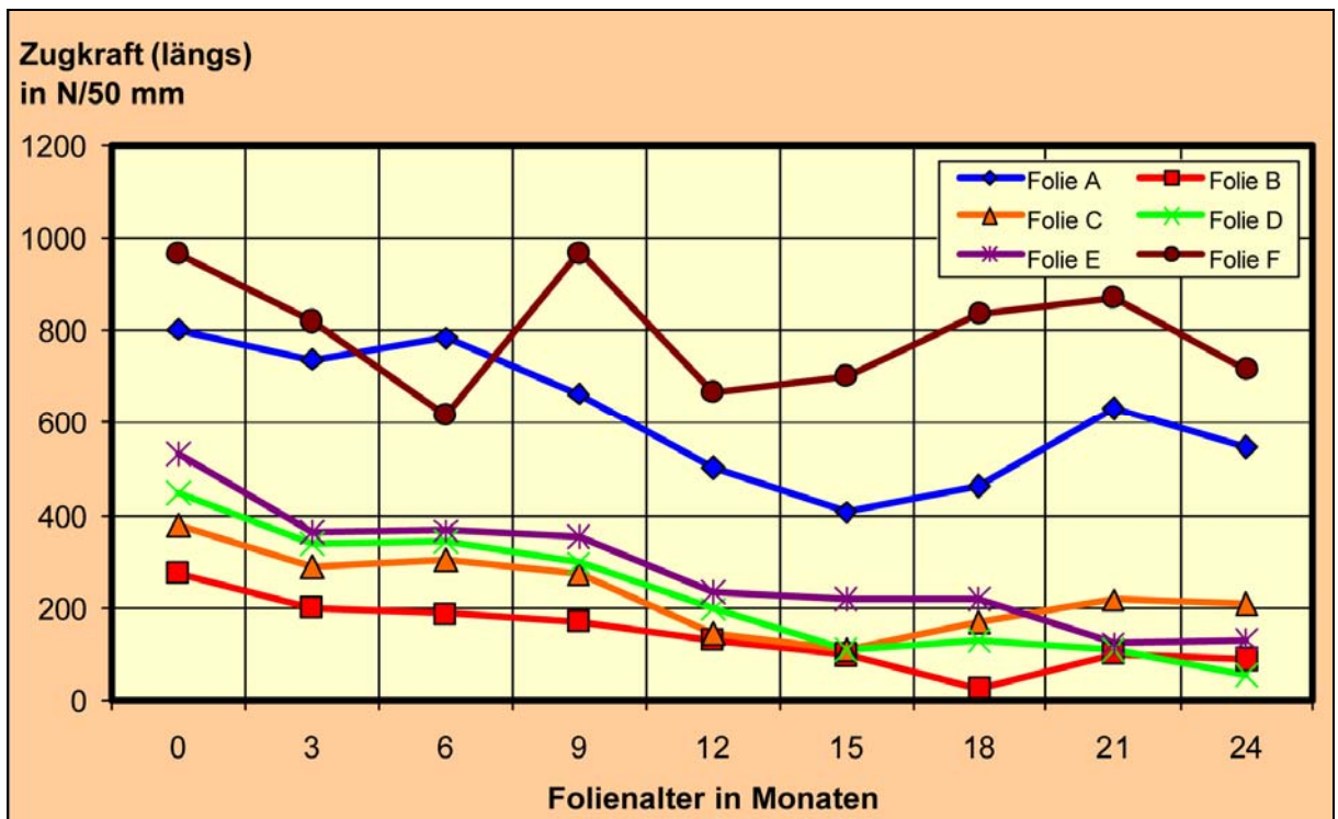
Abb. 17: Zugfestigkeit natürlich gealterter Unterspannbahnen (Folienlängsrichtung)
