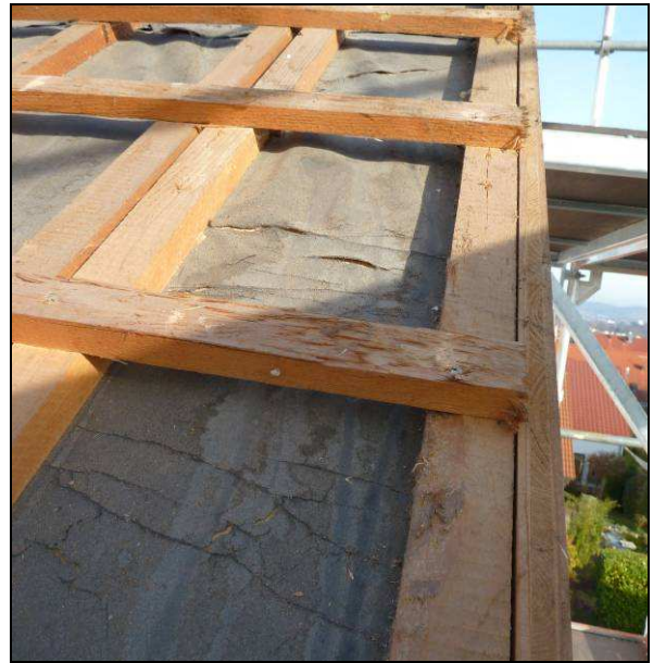
Abb. 45 und 46: o. g. Dachfläche im Bereich von First und Ortgang
