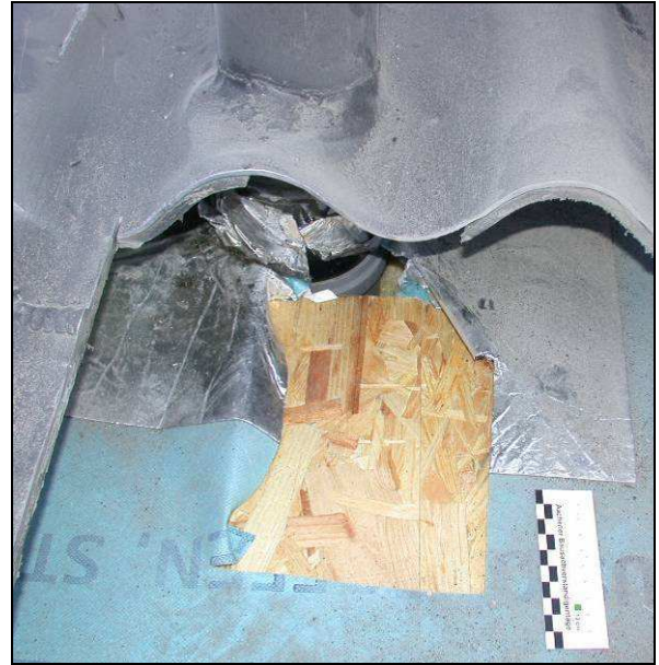
Abb. 52: OSB-Platte war nicht durch Feuchtigkeit geschädigt
