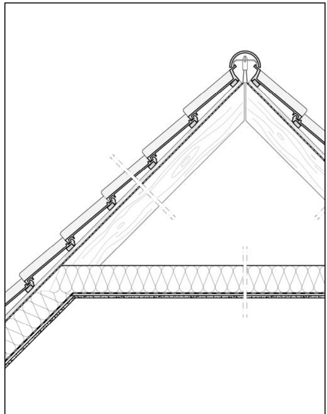
Abb. 8: Übergang zwischen ausgebautem und nicht ausgebautem Dachraum
