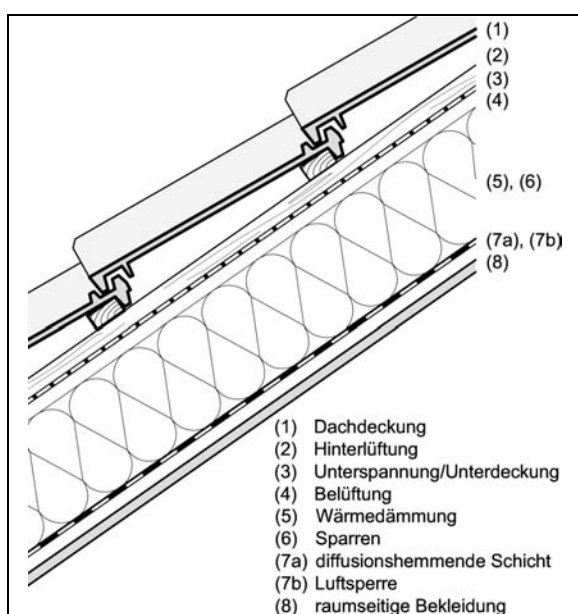
Abb. 1: Belüftete Dachkonstruktion
