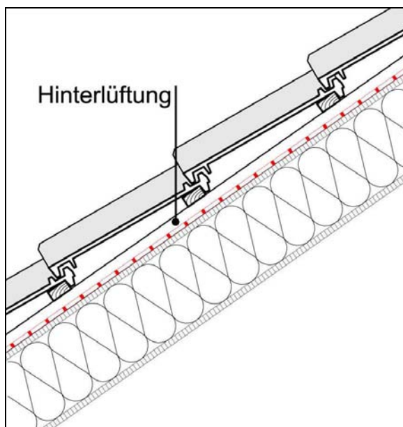
Abb. 9: Unbelüftete Dachkonstruktion, Unterspanbahn auf Schalung verlegt, Vollsparrendämmung
