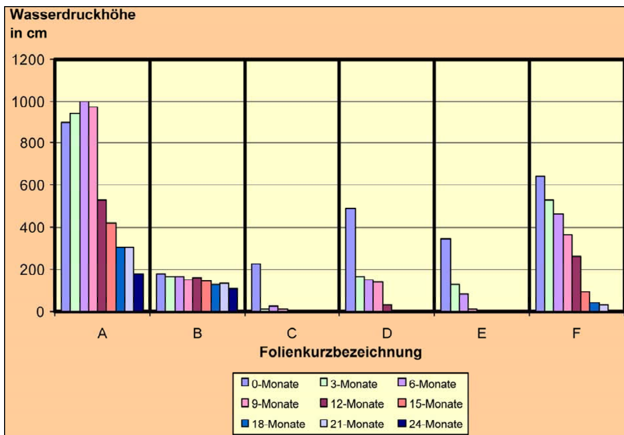
Abb. 13: Wasserdurchdringungswiderstände von frei bewitterten Unterspannbahnen
