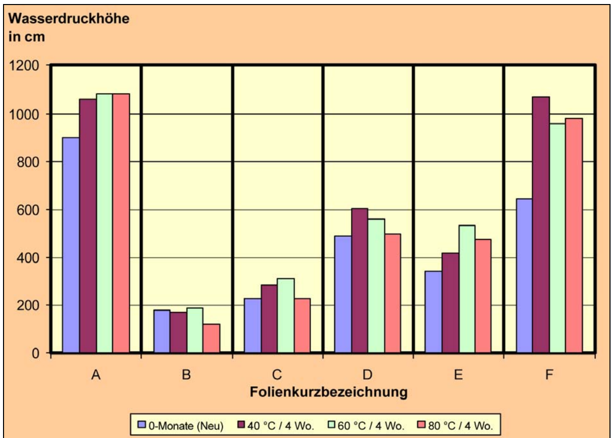
Abb. 14: Wasserdurchdringungswiderstände durch Wärmelagerung künstlich gealterter Unterspannbahnen
