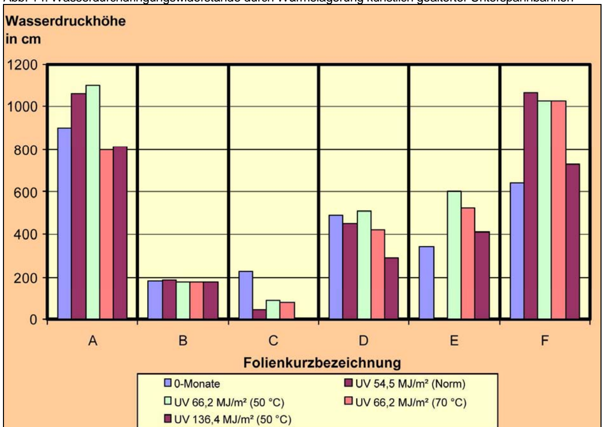
Abb. 15: Wasserdurchdringungswiderstände von durch UV-Bestrahlung künstlich gealterter Unterspannbahnen
