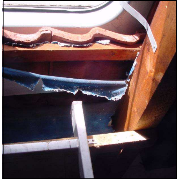
Abb. 30: Schäden am Übergang zur Dachluke
