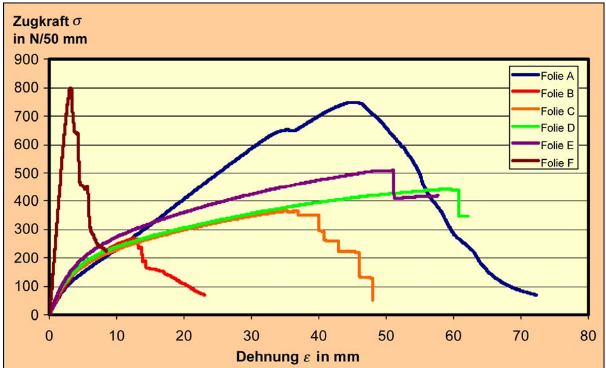
Abb. 16: Zug-Dehnungsdiagramm neuer Unterspannbahnen (Folienlängsrichtung)
