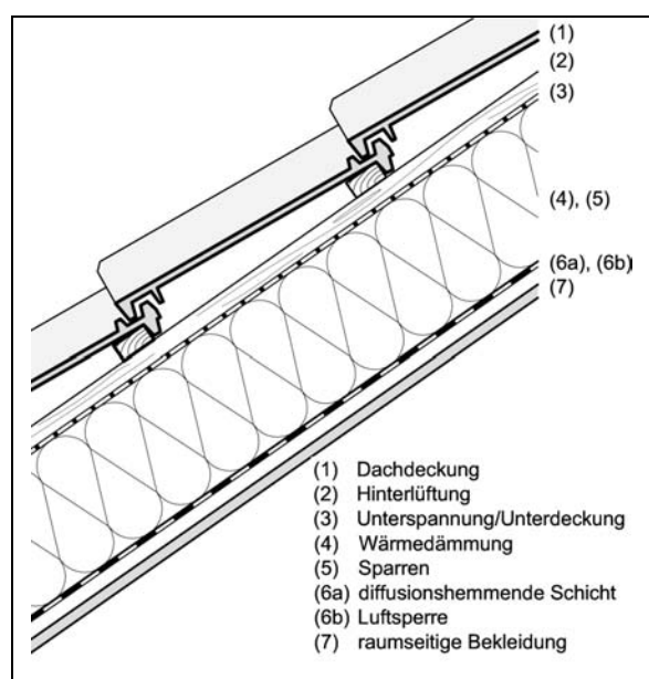
Abb. 2: Unbelüftete Dachkonstruktion
