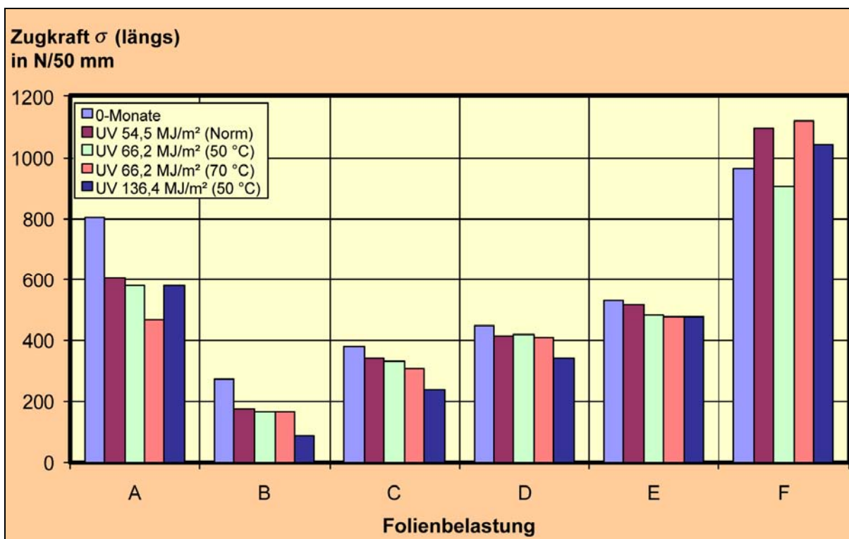
Abb. 19: Zugfestigkeit künstlich durch UV-Bestrahlung gealterter Unterspanbahnen
