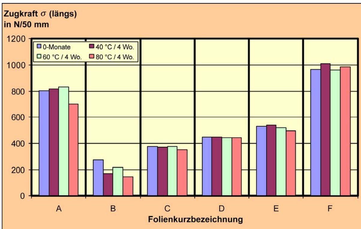
Abb. 18: Zugfestigkeit künstlich durch Wärmelagerung gealterter Unterspanbahnen
