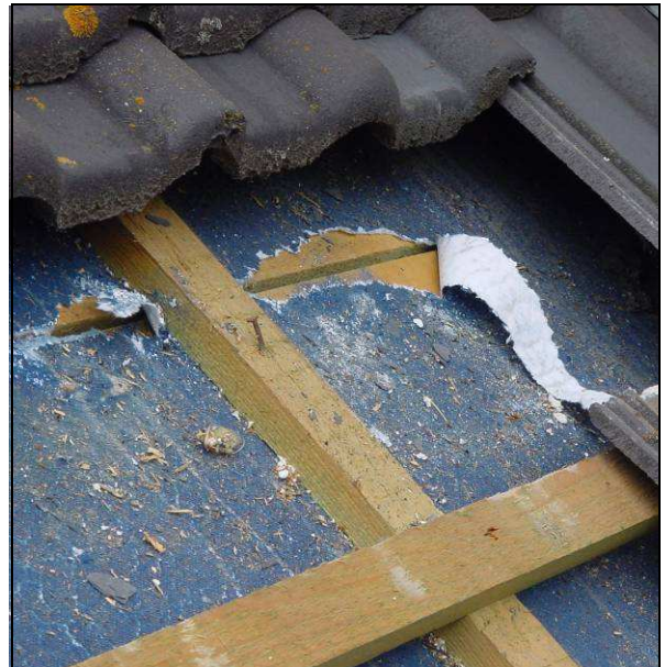
Abb. 31 und 32: Vollständige Zerstörung der Unterspanbahn in der Dachfläche und entlang der Traufe
