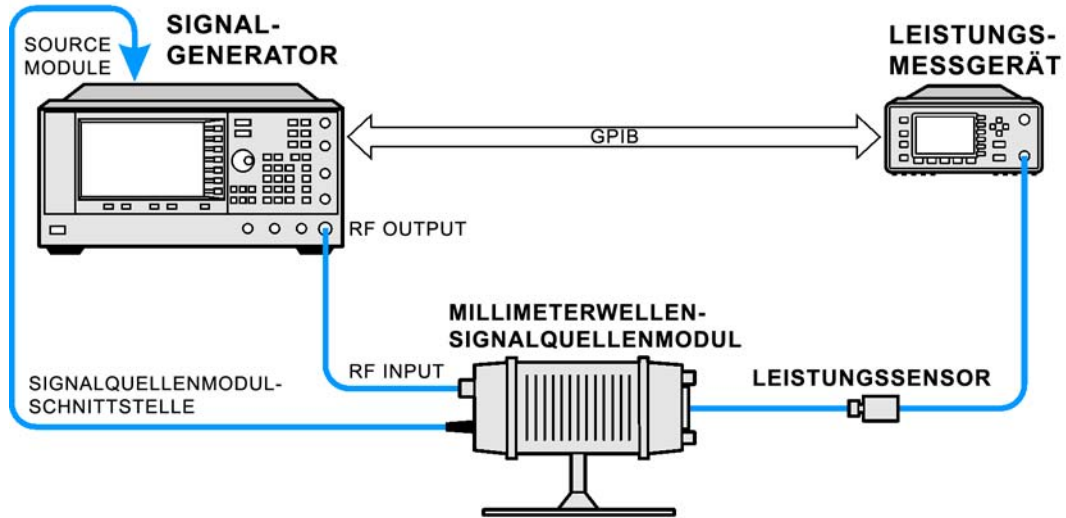
Abbildung 3-6 Benutzerdefinierte Frequenzgangkorrektur für ein Millimeterwellen-Signalquellenmodul in Verbindung mit einem Signalgenerator mit Option 1EA
