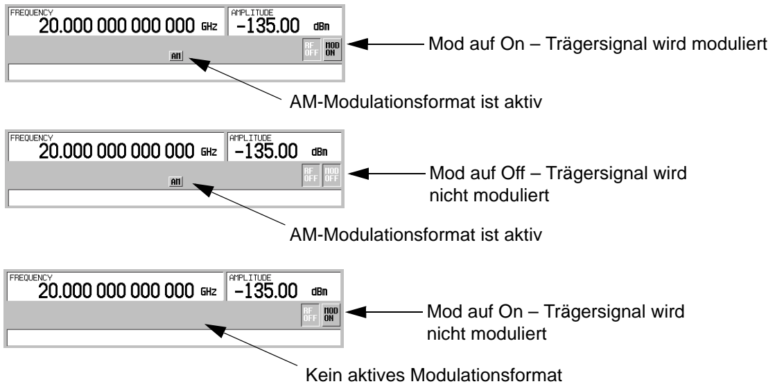
Abbildung 2-10 Modulationsstatus des Trägersignals
