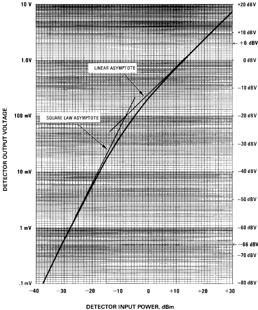
Abbildung 3-3 Typische Diodendetektorkennlinie bei 25° C
