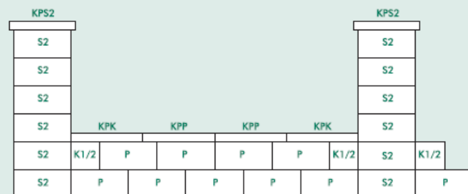
Príklad skladby plotu so stĺpovými tvárniciami S2
