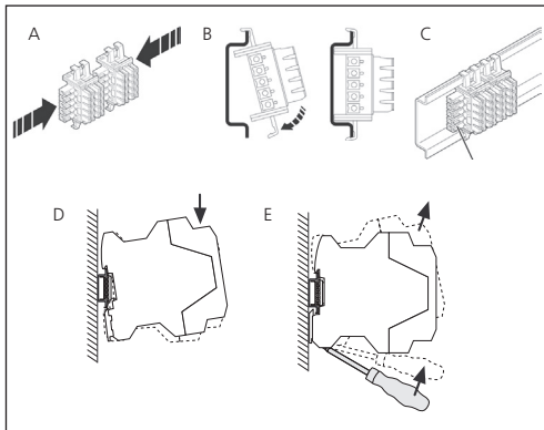
Abb: A Anreihung von Hutschienen-Busverbindern ZU 0628 B Aufrastung von Hutschienen-Busverbindern auf Hutschiene C Hutschienen-Busverbinder auf Hutschiene D Aufrasten eines Meßumformers auf Hutschiene E Entrasten eines Meßumformers von der Hutschiene
