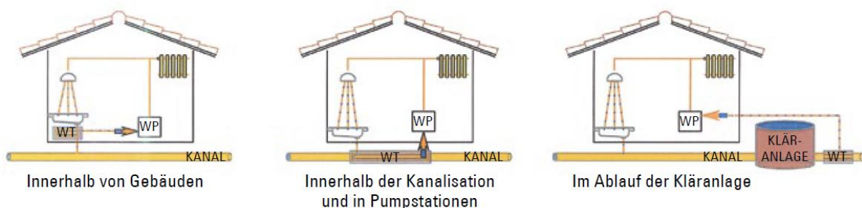
Abbildung 25: Varianten der Abwärmennutzung aus Abwasser (LfU 2015, S. 8)
