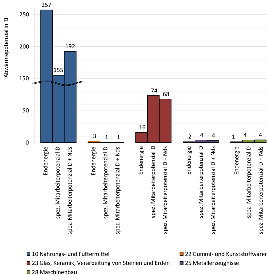
Abbildung 18: Vergleich der jährlichen theoretischen Abwärmepotenziale im Landkreis Cloppenburg auf Basis unterschiedlicher Berechnungsgrundlagen
