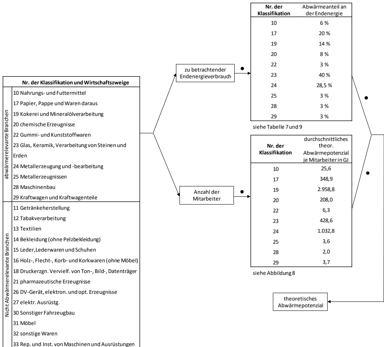
Abbildung 23: Grafische Darstellung der Vorgehensweise zur Ermittlung von theoretischen Abwärmepotenzialen
