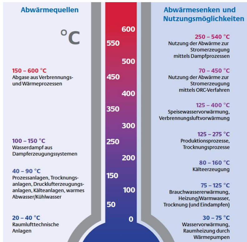
Abbildung 12: Temperaturniveaus verschiedener Abwärmequellen und -senken (Grah, Joest und Raulien 2014, S. 4 f.)
