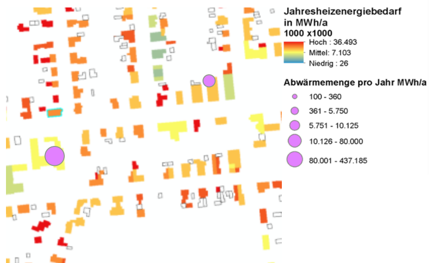
Abbildung 21: Gebäudescharfe Darstellung der tatsächlichen Abwärmepotenziale und der Wärmebedarfe (IP SYSCON GmbH und Landkreis Osnabrück 2017)
