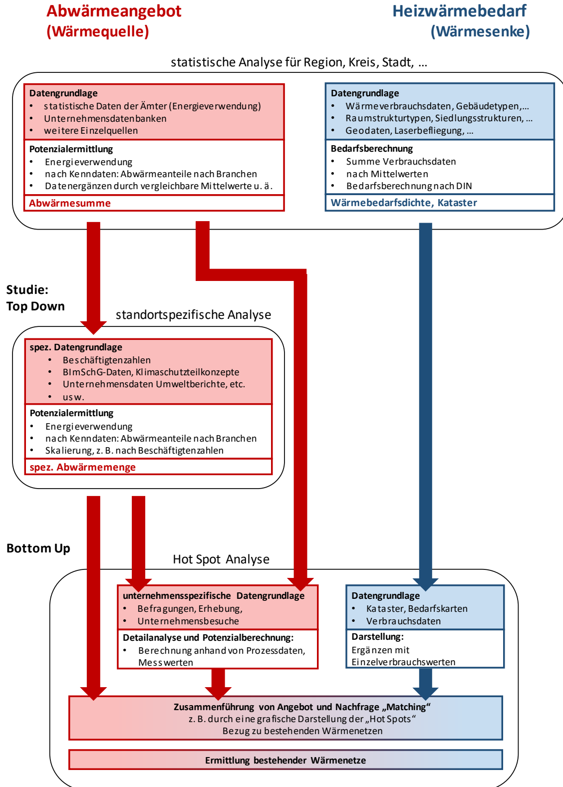
Abbildung 9: Schematische Darstellung der Vorgehensweise zur Erhebung von theoretischen Abwärmepotenzialen
