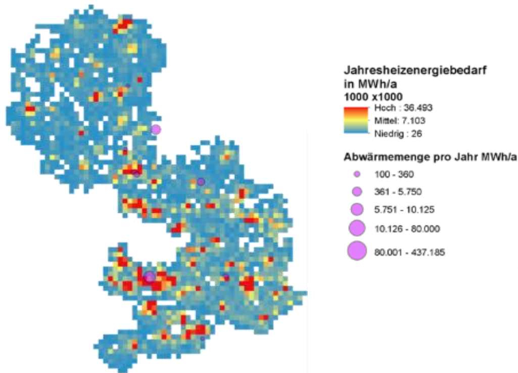
Abbildung 20: Darstellung der tatsächlichen Abwärmepotenziale und Wärmebedarfe für den gesamten Landkreis Osnabrück nach PlnA (IP SYSCON GmbH und Landkreis Osnabrück 2017)
