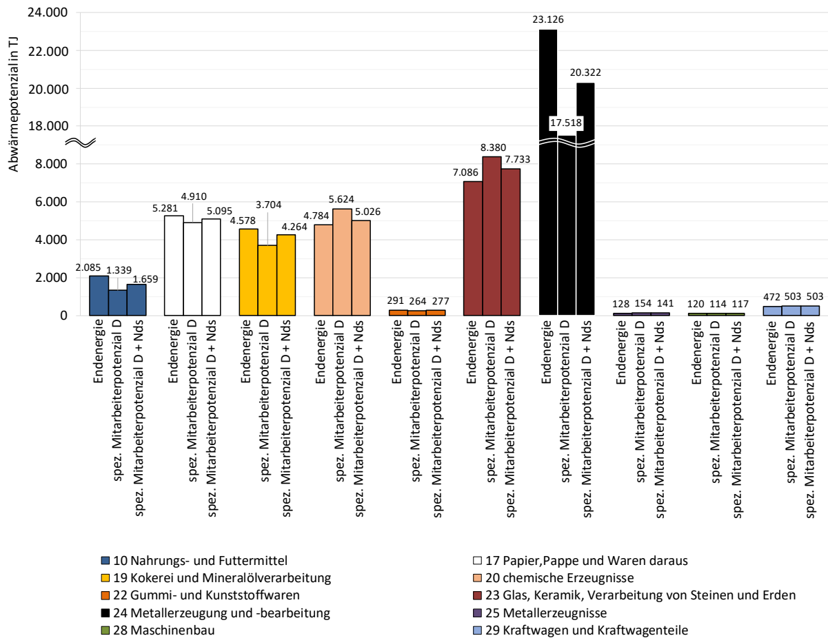
Abbildung 14: Vergleich der jährlichen theoretischen Abwärmepotenziale in Niedersachsen auf Basis unterschiedlicher Berechnungsgrundlagen
