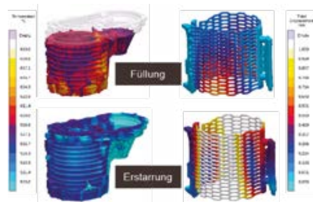
Deformation von Sandkernen über Formfüllung und Erstarrung
