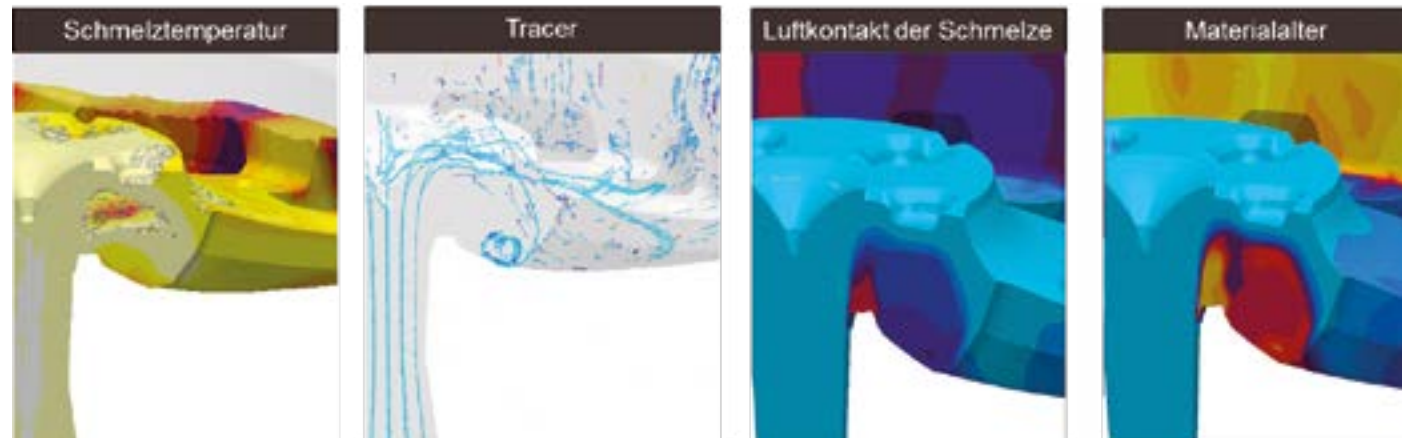
MAGMASOFT®-Ergebnisse zur Formfüllung und Analyse potentieller Gussdefekte wie Kaltlauf oder Oxideinschlüsse
