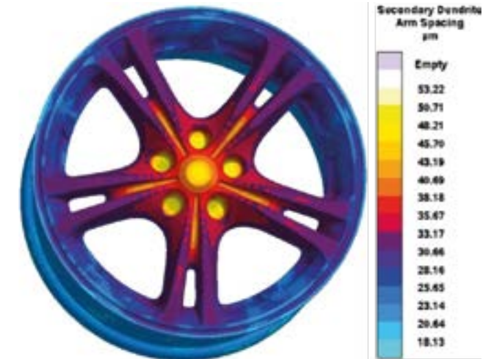
Berechneter lokaler sekundärer Dendritenarmabstand
