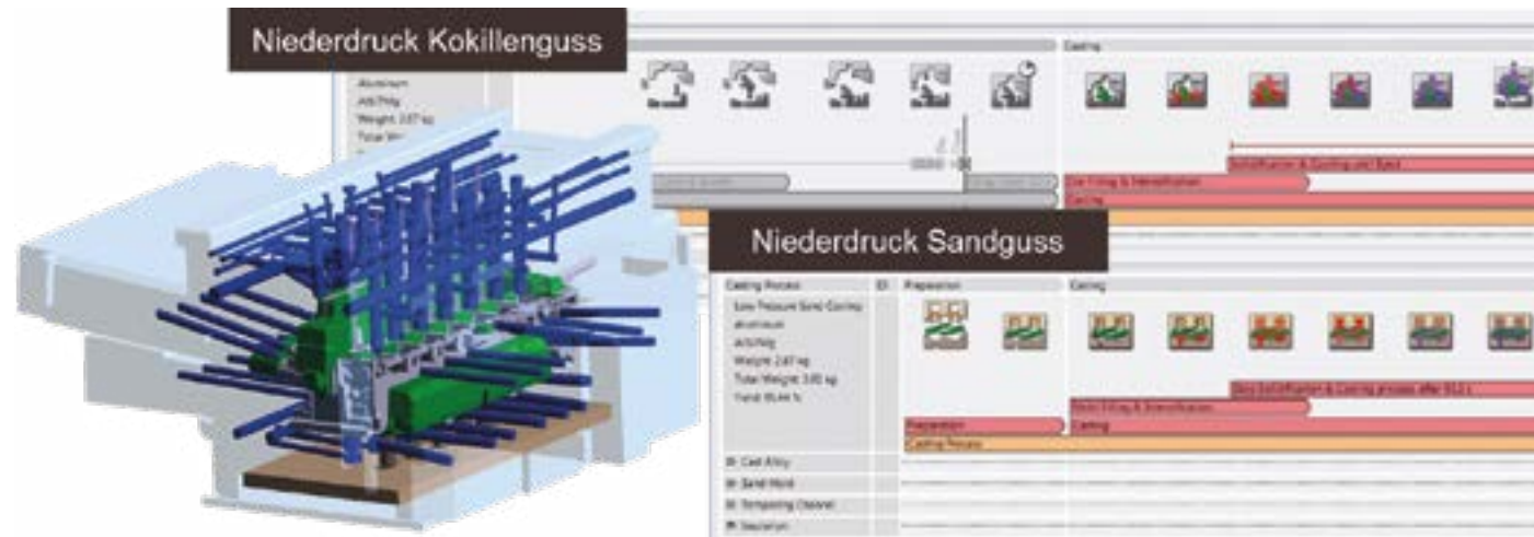
Intuitive verfahrensspezifische Prozessschaubilder für Niederdruck Kokillen- und Sandguss
