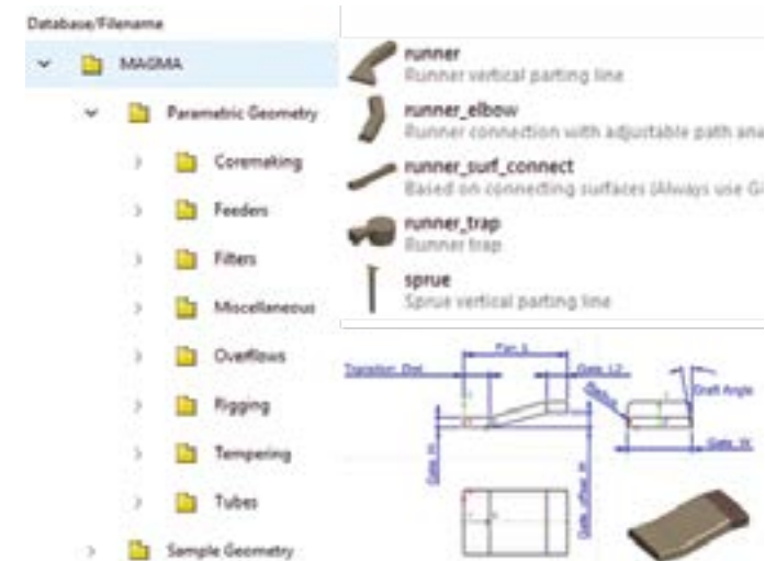
Umfangreiche Datenbank mit voll parametrischen Geometrien für alle wesentlichen Elemente des Kokillengießprozesses
