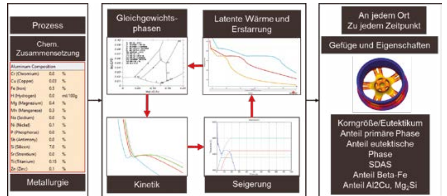
Berechnungszyklus zur Vorhersage der lokalen Gefügestruktur und resultierenden mechanischen Eigenschaften
