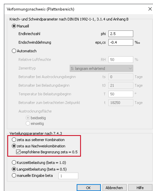
Bild 5. Mindestwert \zeta=0,5 berücksichtigen
