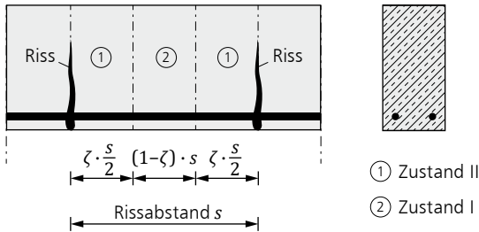
Bild 1. Berechnungsmodell für die Überlagerung der Zustände I und II nach Litzner [3]
