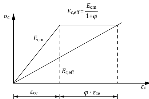
Bild 3. Definition des effektiven E-Moduls unter Berücksichtigung des Kriechens
