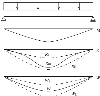
Bild 2. Biegemoment, Krümmung und Verformung eines Stahlbetonbauteils
