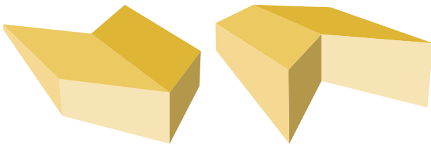
Bild 10. Beispiele für polygonale Kontaktflächen von Grat- und Kehlsparren mit den Pfetten – die einzelnen Flächenanteile sind verschiedenfarbig dargestellt
