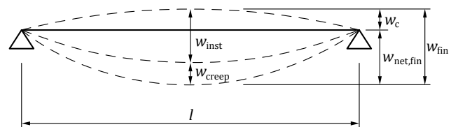
Bild 8. Anteile der Durchbiegung [1]
