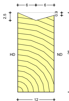
Bild 7. Sparren mit Kehlausbildung
