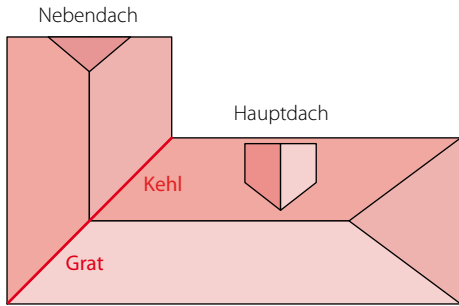
Bild 1. Dachskizze
