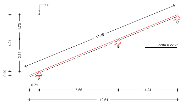
Bild 3. Lasteinzugsflächen des Sparrens
