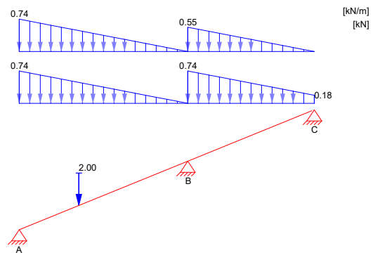
Bild 6. Grafische Ausgabe der Belastung je Einwirkung
