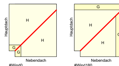
Bild 4. Ausgabe der Windbereiche
