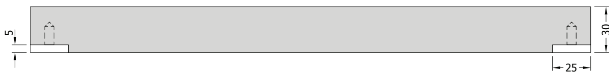
Längsschnitt
