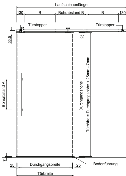
Schiebetür mit eingesetztem Beschlag
