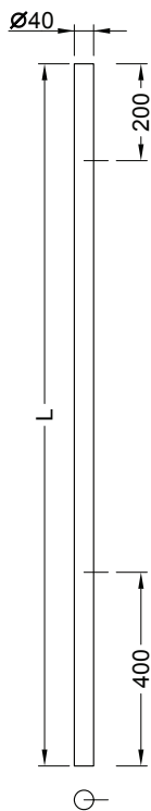
Typ A Endsäule
