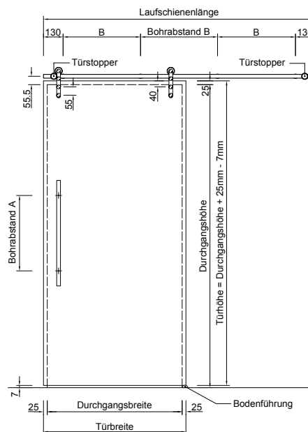
Schiebetür mit aufgesetztem Beschlag
