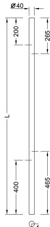
Typ E Drehsäule versetzt
