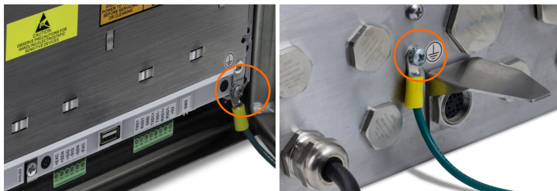
Figure 2-5: Points de mise à la terre du terminal IND570xx avec montage sur panneau (à gauche) et pour environnement rude (à droite)
