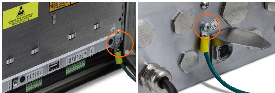
Abbildung 2-5: Erdungspunkte, IND570xx-Terminal für den Schaltschrank-Einbau (links) und mit Gehäuse für raue Umgebungen (rechts)
