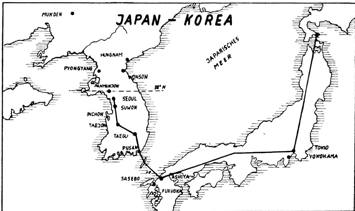
Fig. 16. Richtstrahlachsen der 8. Armee Japan - Korea
