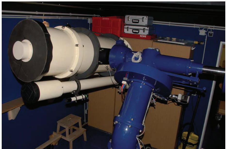
Abb. 2: Das 12,5"-Newton-Cassegrain-Teleskop neben dem 110mm-Achromat-Refraktor auf der schweren Zeiss-Montierung
