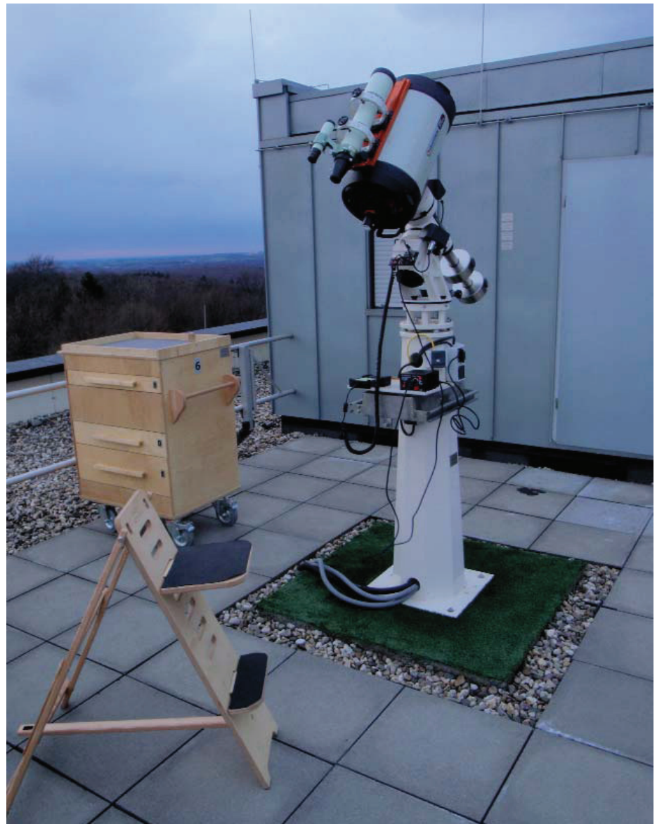
Abb. 5: Nach wenigen Handgriffen ist das Teleskop auf die Montierung gesetzt. Strom- und EDV-Anschlüsse sind vorhanden und sofort benutzbar.
