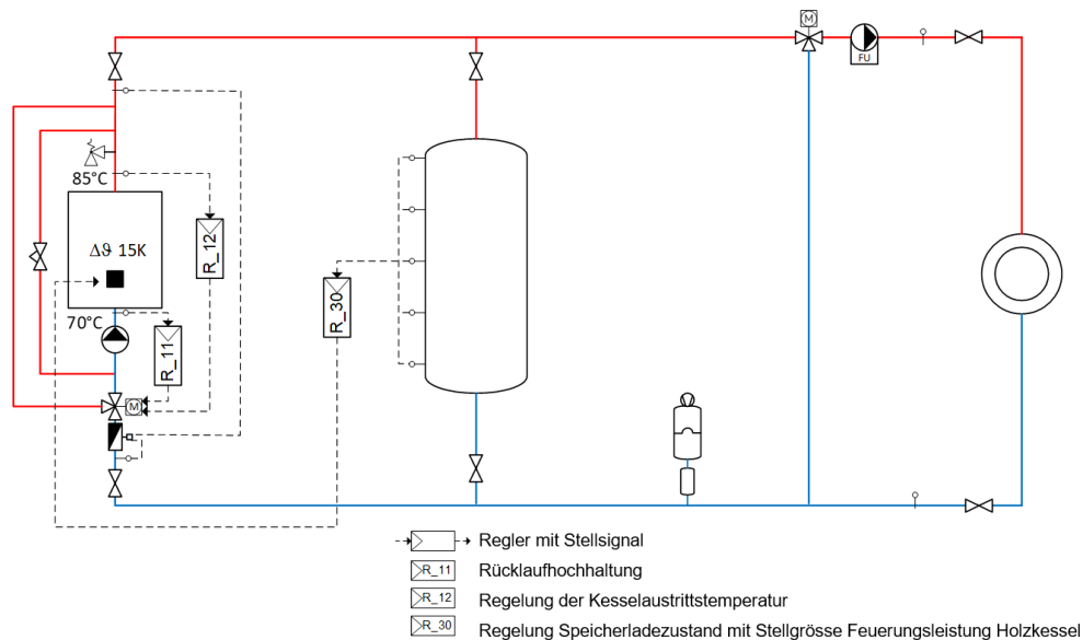
Bild 7.14 Regelung des Speicherladezustands mit Stellgröße Feuerungsleistung Holzkessel.
