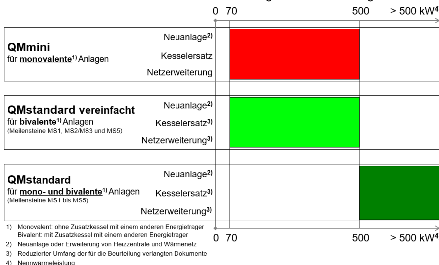
Bild 2.1 Anwendungsbereich von QMstandard® und QMmini® in der Schweiz.
