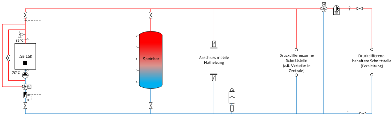
Bild 13.6 Prinzipschema einer Anlage mit einem Holzkessel mit Speicher (WE2).
