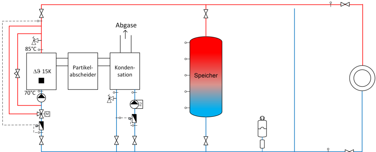
Bild 13.18 Prinzipschema einer Anlage mit Einbindung der Abgaskondensation in den Haupt-Rücklauf: Abgaskondensations-Eintritt und Abgaskondensations-Austritt zwischen Speicher und Kessel.
