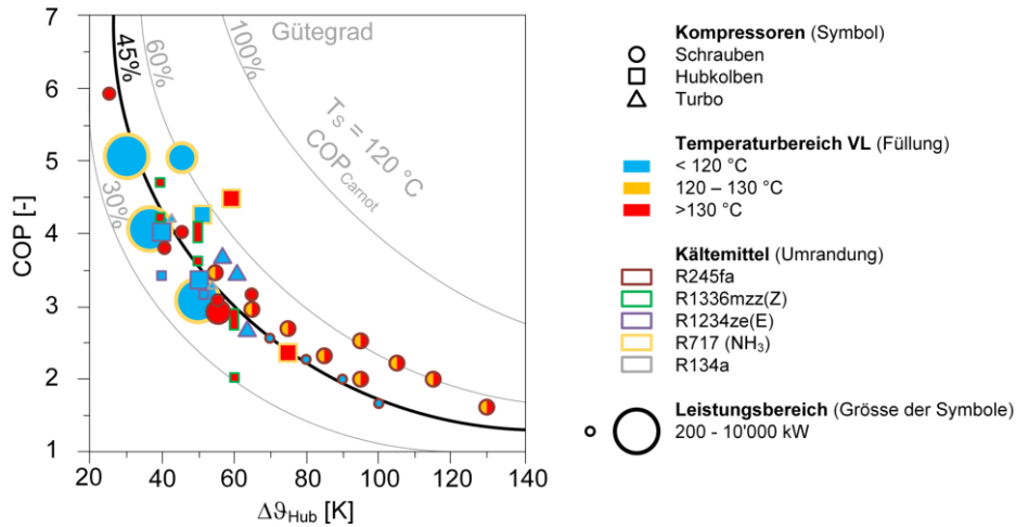
Bild 13.23 Gütegrad und COP realer Maschinen in Abhängigkeit des äusseren Temperaturhubes, der Temperaturdifferenz zwischen Senkenaustritts- und Quelleneintrittstempertur (selbst gezeichnet auf Basis von [134]).
