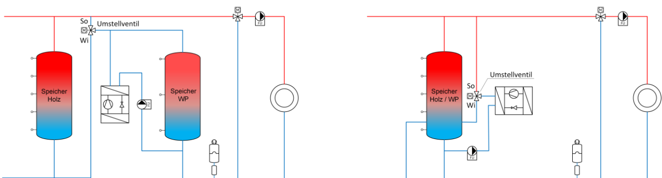
Bild 13.24 Prinzipschema zur Einbindung einer Wärmepumpe für den Sommerbetrieb.
