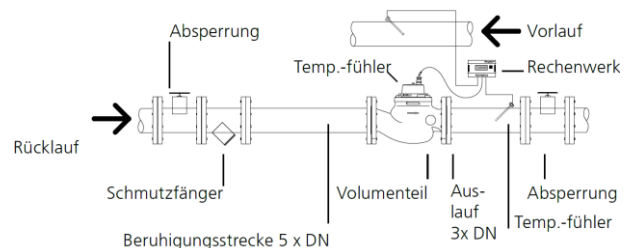
Bild 7.10 Installation Wärmehäher (Quelle: WDV-Molliné GmbH).
