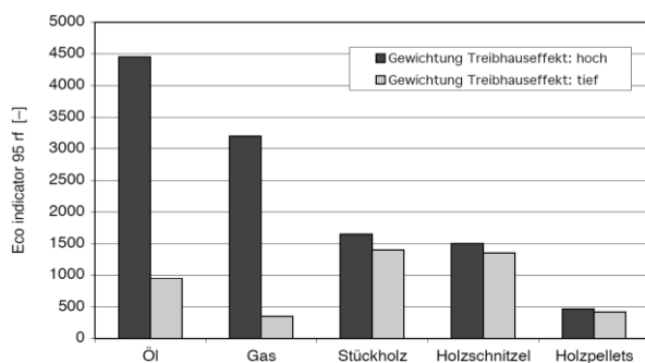
Bild 13.1 Umweltbelastung als Eco-Indikator-Punkte pro TJ Nutzenergie für Öl-, Gas- und Holzheizungen für die Gewichtungsvarianten des Treibhauseffekts «hoch» und «tief» nach Daten von [132].
