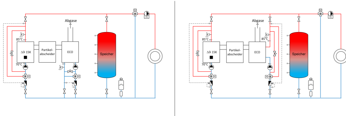
Bild 13.16 Prinzipschema einer Anlage mit der Einbindung eines Economisers in Serie im Rücklauf (links) oder parallel (rechts).
