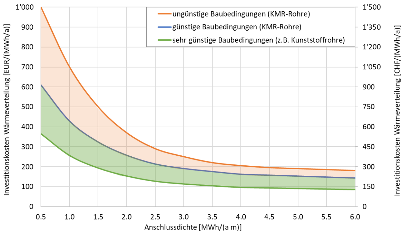
Bild 10.9 Spezifische Investitionskosten Wärmeverteilung – Auswertung realisierter Anlagen aus AT und CH im Zeitraum 2009 - 2018. In den Kosten enthalten sind die Fernleitungsgruppe in der Heizzentrale, das Fernleitungsnetz inklusive Grabarbeiten sowie die Hausanschlüsse bis und mit Wärmeübergabestationen (ohne Hauszentrale); EUR/CHF - Umrechnung berücksichtigt unterschiedliche Preisniveaus in AT und CH.
