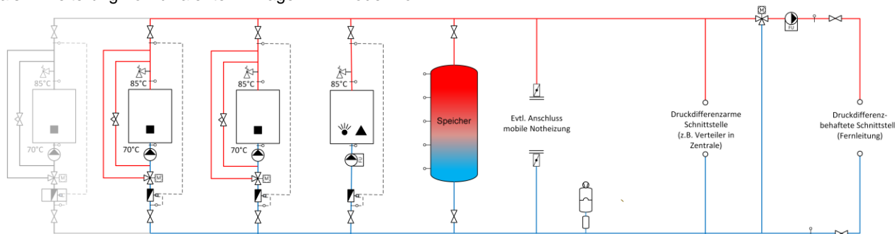
Bild 13.10 Prinzipschema einer Anlage mit zwei Holzkesseln mit Speicher und fossilem Kessel (WE8).
