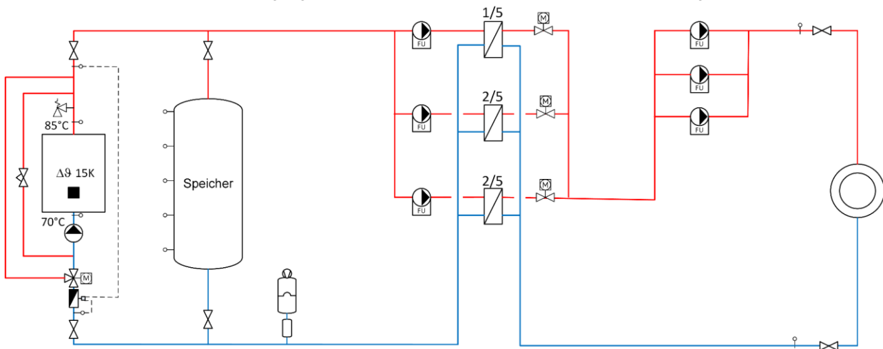
Bild 7.21 Netztrennung Wärmeerzeugung/Fernwärmenetz mit drei Wärmeübertrager.
