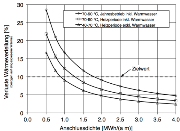
Bild 12.3 Wärmeverteilverluste in Funktion der Anschlussdichte für verschiedene Betriebsweisen und Vorlauftemperatur-Niveaus des Wärmenetzes.
