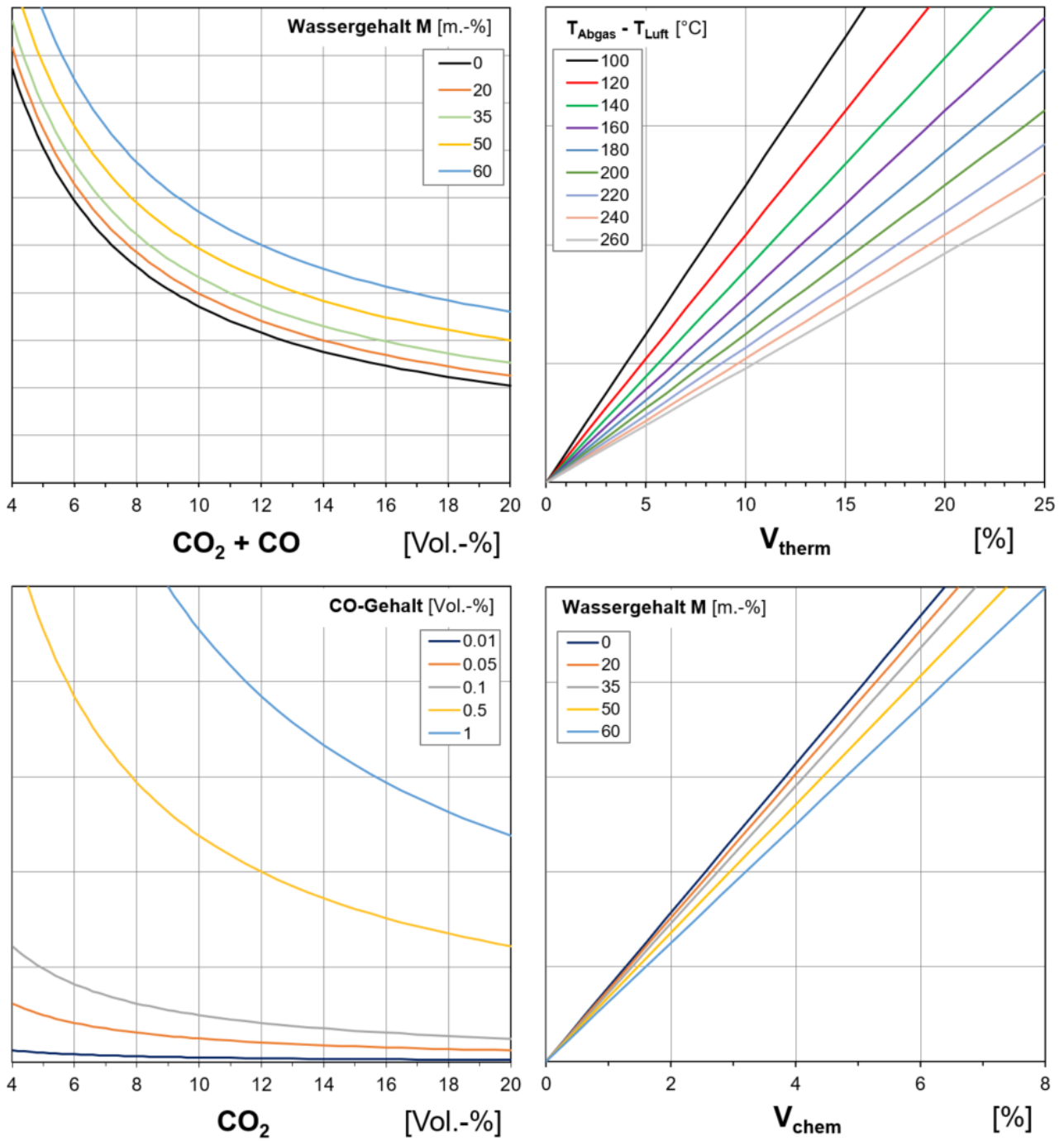
Bild 20.8 Nomogramme zur Bestimmung des feuerungstechnischen Wirkungsgrads mit \eta_f = 100 - V_{therm} - V_{chem} [%]
