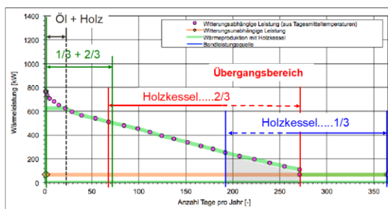
Bild 13.5 Betriebsphasen und Übergangsbereich bei Anlagen mit zwei Holzkesseeln am Beispiel der Jahresdauerlinie (links mit fossilem Kessel, rechts ohne fossilen Kessel).
