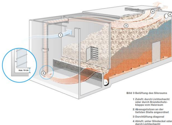
Bild 14.3 Silobelüftung (Quelle: Suva [138]).
