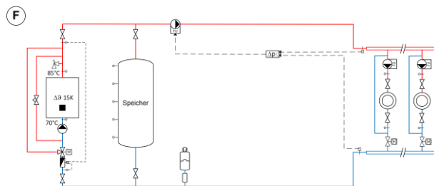
Bild 7.20 Hydraulische Einbindung Wärmespeicher – Schaltung F.
