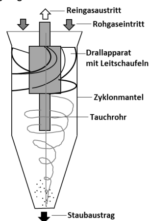
Bild 5.15 Schnitt durch einen Einzelzyklon (Axialabscheider).
