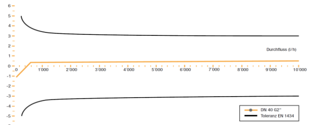
Bild 7.9 Fehlerkurve Schwingstrahl Durchflussmessverfahren (Quelle: NeoVac Superstatic 440).
