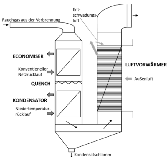
Bild 5.22 Schema einer Abgaskondensationsanlage.
