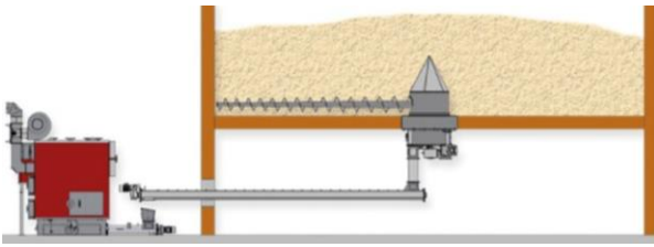
Bild 6.23 Austragungssystem mit Zentrumschnecke (Quelle: Binder Energietechnik GmbH, Siloentnahmeschnecke Type SES-E1L von-Gottwald GmbH Maschinenbau).
