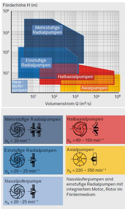
Bild 7.4 Typologie von Pumpen nach Förderhöhe und Volumenstrom [72].
