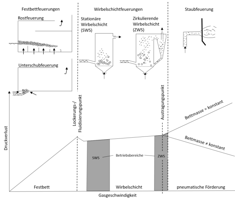
Bild 5.3 Übersicht Feuerungstechnologien. Einteilung nach Strömungsgeschwindigkeit des Brenngases durch die Anlage und Art des Brennstofftransports.
