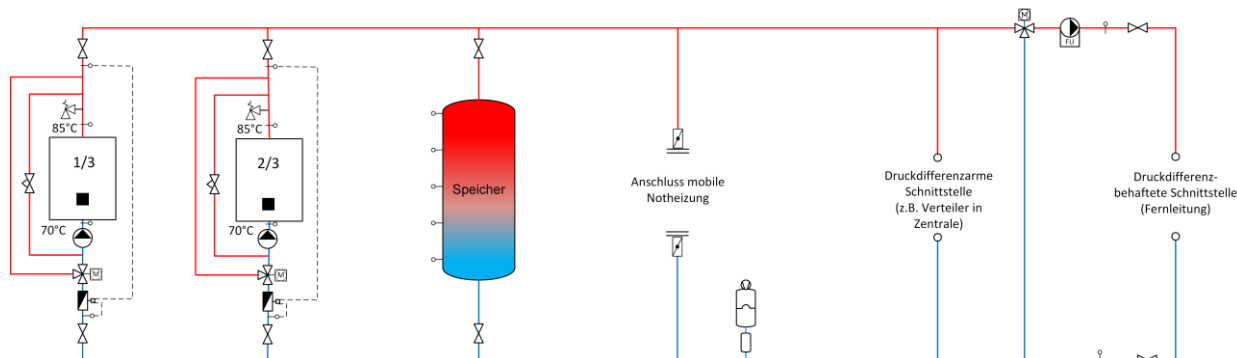
Bild 13.8 Prinzipschema einer Anlage mit zwei Holz-kesseln und mit Speicher (WE6).
