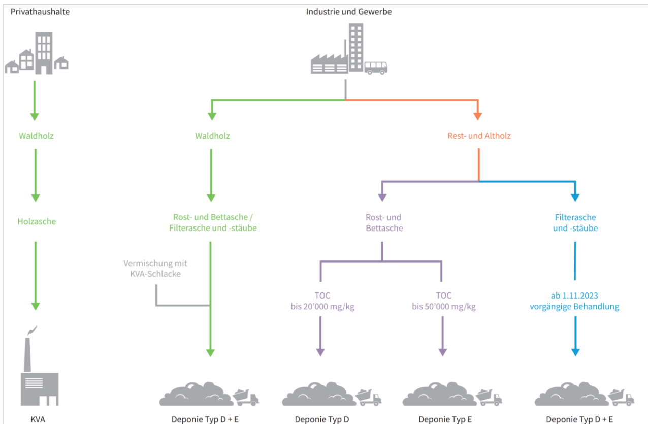
Bild 9.3 Entsorgungspfade in der Schweiz (KVA ... Kehrlichtverbrennungsanlage, TOC ... gesamter organische Kohlenstoff, Deponietypen entsprechend Schweizer Abfallverordnung) [89].
