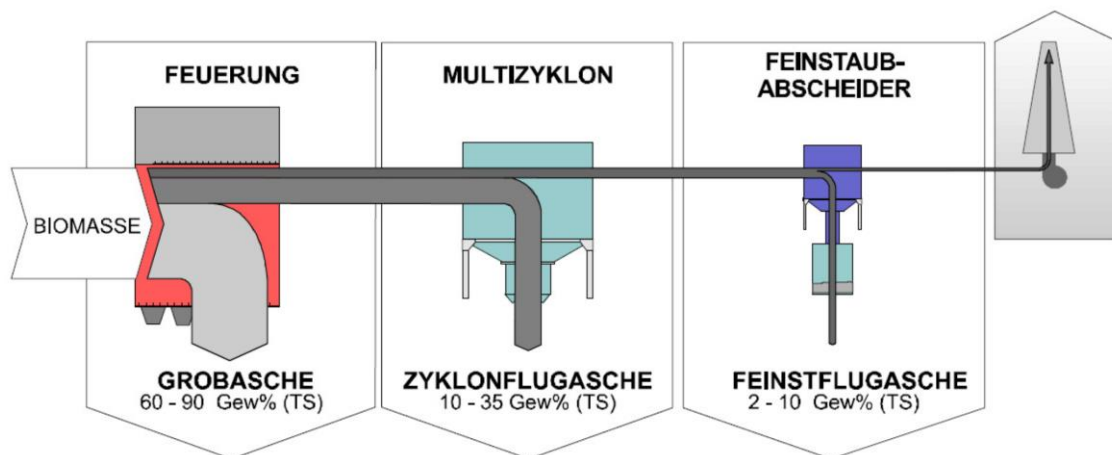
Bild 9.1 Anteile der verschiedenen Aschefraktionen in Gewichtsprozent (Trockensubstanz TS) [81].
