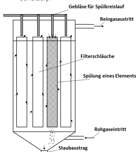
Bild 5.16 Schema eines Gewebefilters: Parallele Anordnung der Filterschlauch-Elemente. Jeweils drei Elemente sind in Arbeitsposition, das vierte Element wird im Gegenstrom-Prinzip gereinigt (Abreinigung mit Druckluft).
