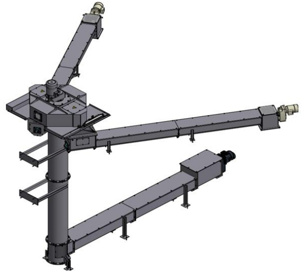
Bild 6.31 Schneckenförderer horizontal bis vertikal fördernd (Quelle: Schmid energy solutions).
