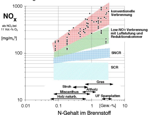
Bild 13.29 Vergleich der NO x -Emissionen in Abhängigkeit der unterschiedlichen Stickstoffgehalte im Brennstoff bei unterschiedlichen Reduktionsmassnahmen [120].
