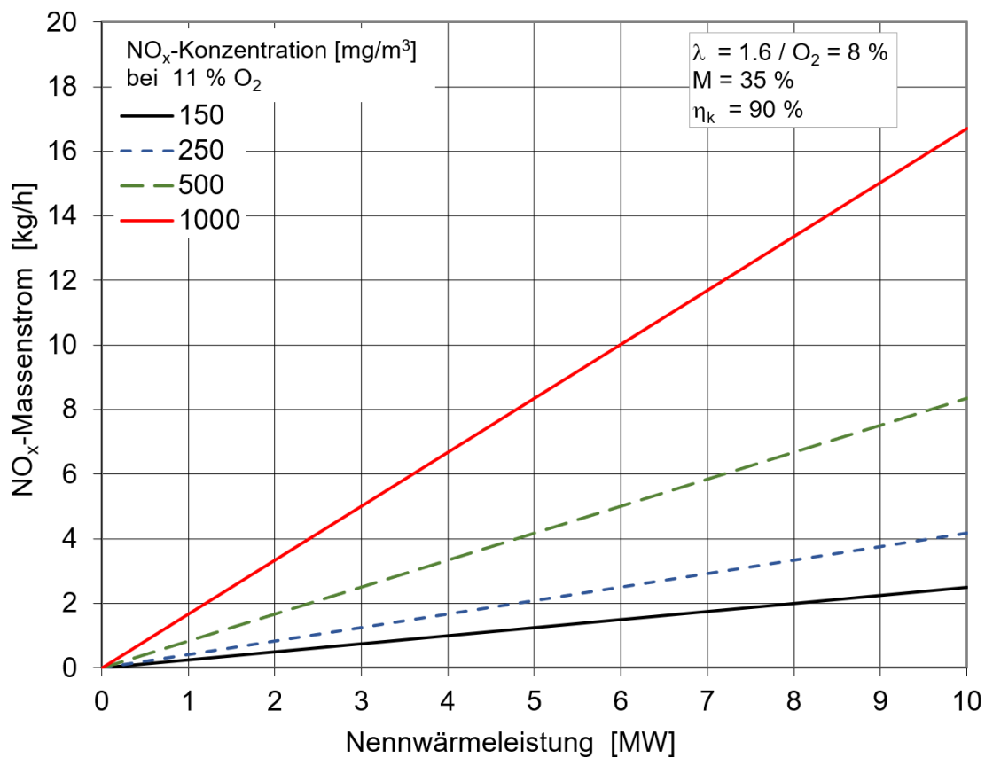
Bild 20.7 NO x -Massenstrom in kg/h in Funktion der Nennwärmeleistung in MW und verschiedener NO x -Konzentrationen.
