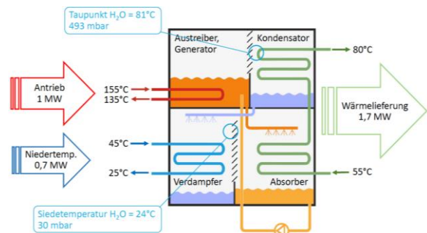
Bild 13.26 Absorbtionswärmepumpe (LiBr, einstufig; Quelle: STEPSAHEAD).
