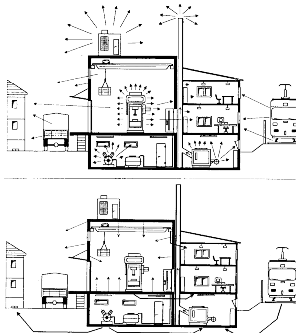
Bild 13.34 Luft- und Körperschall [68].
