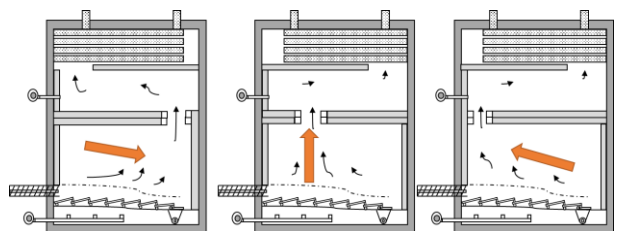
Bild 5.7 Bauprinzipien von Rostfeuerungen; Gleichstrom (links), Mittelstrom (mitte) und Gegenstrom (rechts).
