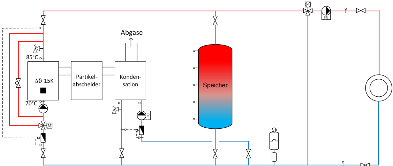
Bild 13.17 Prinzipschema einer Anlage mit Einbindung der Abgaskondensation in den Haupt-Rücklauf: Abgaskondensations-Eintritt vor dem Speicher, Abgaskondensations-Austritt zwischen Speicher und Kessel.
