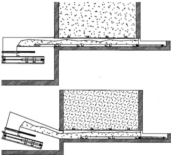
Bild 6.32 Schubsystem horizontal fördernd (oben) und steigend fördernd (unten) [68].
