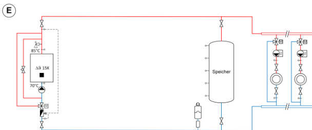
Bild 7.19 Hydraulische Einbindung Wärmespeicher – Schaltung E.
