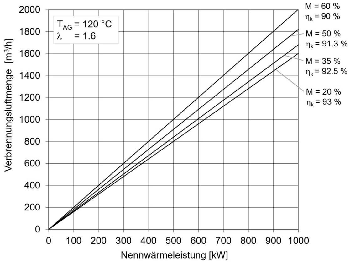
Bild 20.4 Verbrennungsluftmenge in Funktion von Nennwärmeleistung und Wassergehalt
