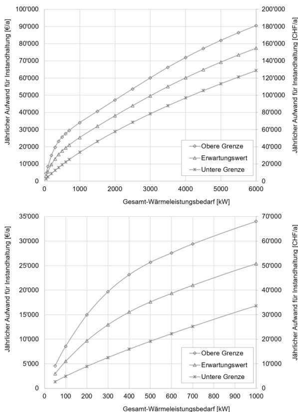
Bild 17.1 Jährlicher Aufwand für Instandhaltung in Abhängigkeit des Gesamt-Wärmeleistungsbedarfs der Anlage (Erfahrungswert = 4 % der Investkosten gemäss Bild 10.8). Oben: Bereich bis 6'000 kW Unten: Bereich bis 1'000 kW.
