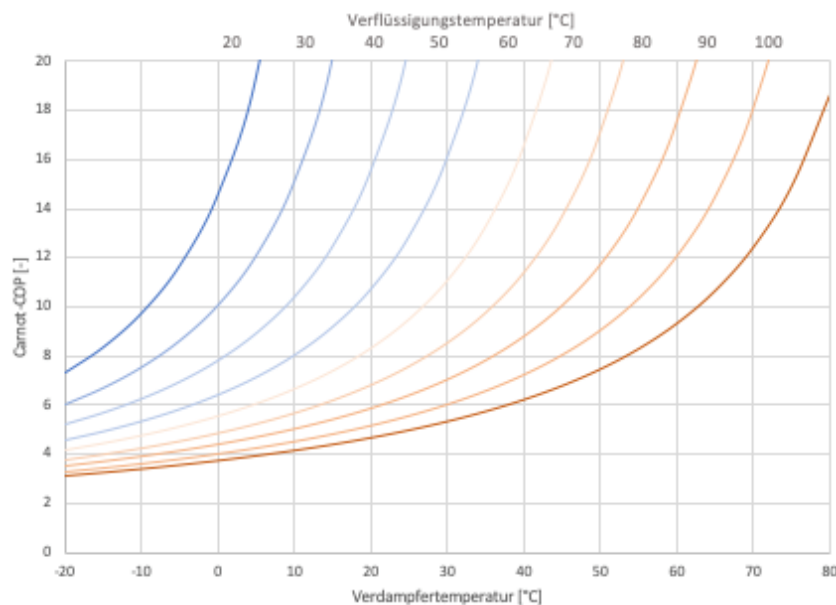
Bild 13.22 COP des Carnot-Prozesses. Das Diagramm basiert auf einem Gütegrad von 1 einer idealen Maschine respektive Wärmepumpe. Wärmepumpen weisen im Realbetrieb einen Gütegrad von 0.4 bis 0.6 auf.
