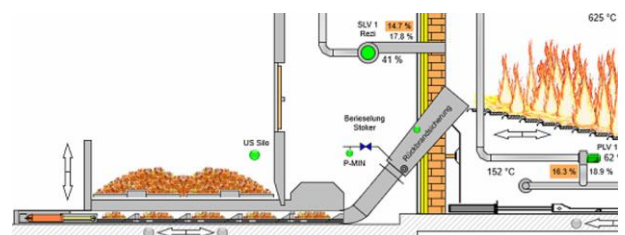
Bild 6.37 Beschickung mit Direkteinschieber (Quelle: Agro Forst & Energietechnik GmbH).
