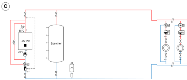
Bild 7.17 Hydraulische Einbindung Wärmespeicher – Schaltung C.
