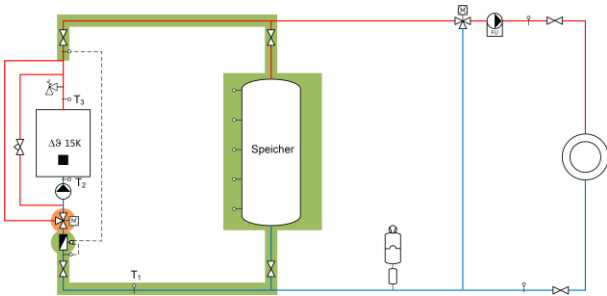
Bild 7.1 Kesselkreis mit konstantem Durchfluss und der Strecke mit variablem Durchfluss in grün.
