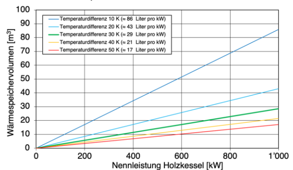
Bild 7.11 Volumen des Wärmespeichers in Funktion der Kesselnennleistung und der Temperaturdifferenz.
