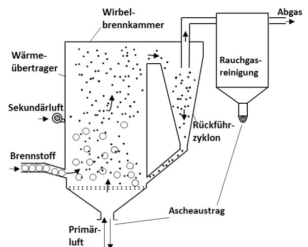
Bild 5.8 Funktionsprinzip einer zirkulierenden Wirbelschichtfeuerung.
