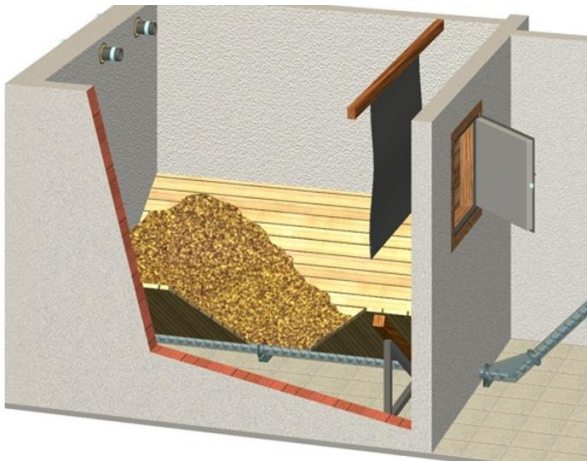
Bild 6.29 Pellet-Austragungssystem mit Schrägboden [68].
