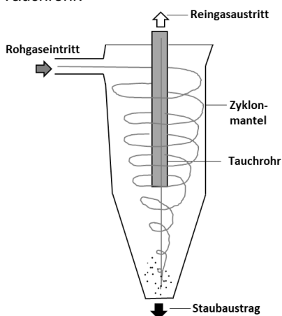
Bild 5.14 Schnitt durch einen Einzelzyklon (Tangentialabscheider).
