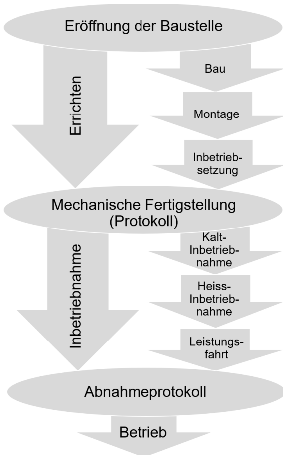
Bild 15.1 Errichten, Inbetriebnahme und Betrieb einer Anlage (auf Basis von [139] selbst erstellt).
