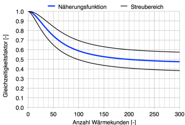
Bild 12.2 Funktion und Streubreich für den Verlauf des Gleichzeitigkeitsfaktors in Abhängigkeit der Anzahl der Wärmekunden/-kunden (siehe [19]).
