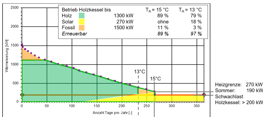
Bild 13.27 Jahresdauerlinie eines Holzheizwerks mit einem Holzkessel, einem fossilen Heizkessel und einer Solarthermieanlage.
