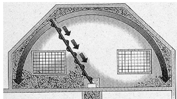
Bild 6.25 Austragungssystem mit Pendelschnecke [68].
