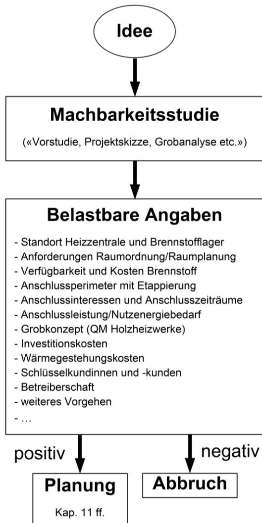
Bild 3.2 Einbindung der Machbarkeitsstudie in die Projektentwicklung.
