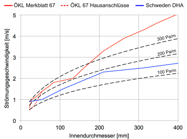
Bild 12.4 Strömungsgeschwindigkeiten in Funktion des Rohrinneendurchmessers mit Empfehlungen für maximale Fließgeschwindigkeit nach ÖKL Merkblatt 67 [101] und der Swedish District Heating Association (DHA) [77]. Zudem sind die Strömungsgeschwindigkeiten bei konstanten spezifischen Druckverlusten von 100, 200 und 300 Pa/m dargestellt [120].
