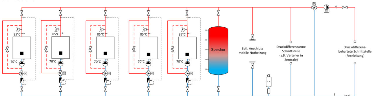
Bild 13.12 Prinzipschema einer Mehrkesselanlage («Kaskadenanlage») mit Standard-Seriengeräten.
