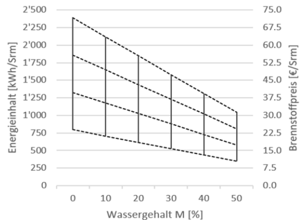
Bild 4.5 Volumenbezogener Energieinhalt und Richtwerte für Brennstoffpreise von Hackschnitzeln in Abhängigkeit des Wassergehalts für Schüttdichten zwischen 150 kg/Srm (unten) und 450 kg/Srm (oben); Berechnungsgrundlage 30 €/MWh.
