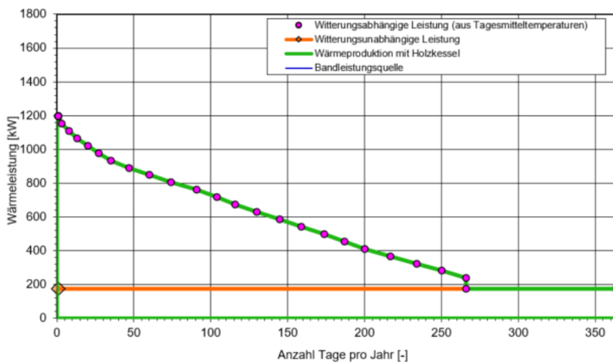
Bild 11.3 Jahresdauerlinie der benötigten Wärmeleistung, grün umrahmt die mit Holz produzierte Jahresenergiemenge.
