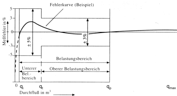
Bild 7.8 Fehlerkurve mechanisches Durchflussmessverfahren mit Flügelrad.
