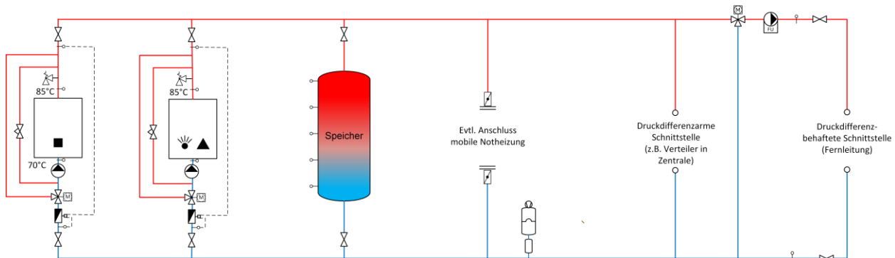
Bild 13.7 Prinzipschema einer Anlage mit einem Holz-kessel mit Speicher und fossilem Heizkessel (WE4).
