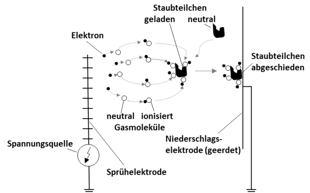
Bild 5.19 Physikalisches Wirkungsprinzip eines Elektroabscheiders.
