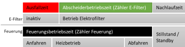
Bild 5.20 Typischer Betriebszyklus einer Feuerung und eines Elektroabscheiders (siehe FAQ 38).
