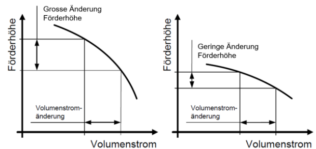
Bild 7.5 Steile (links) und flache Pumpenkennlinie (rechts).
