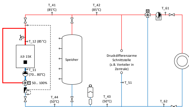
Bild 7.3 Hydraulische Einbindung des Kesselkreises ohne und mit Bypass.
