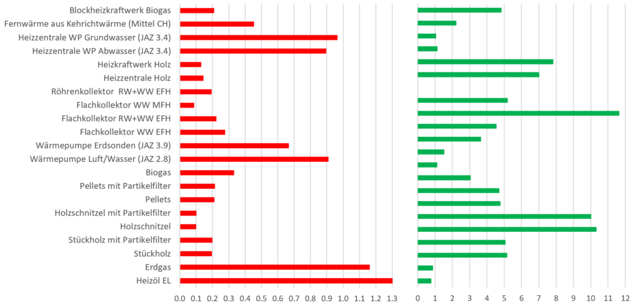
Bild 13.2 Links (rot): Primärenergiefaktor an nichterneuerbarer Energie bez. kumulierter Energieaufwand KE_{NE} Rechts (grün): Erntefaktor an nichterneuerbarer Energie EF_{NE} = 1/KE_{NE} nach Tabelle 13.2
