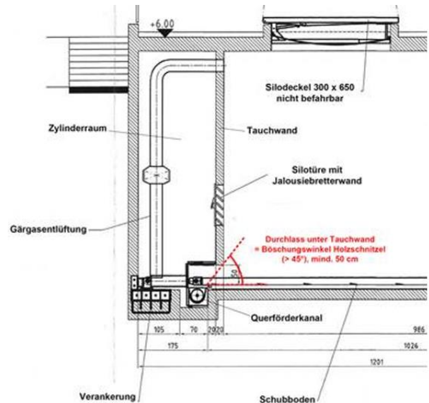
Bild 14.2 Durchlassöffnung vom Silo zum Querböhrerkanal (Quelle: Holzenergie Schweiz).
