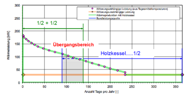
Bild 13.5 Betriebsphasen und Übergangsbereich bei Anlagen mit zwei Holzkesseeln am Beispiel der Jahresdauerlinie (links mit fossilem Kessel, rechts ohne fossilen Kessel).
