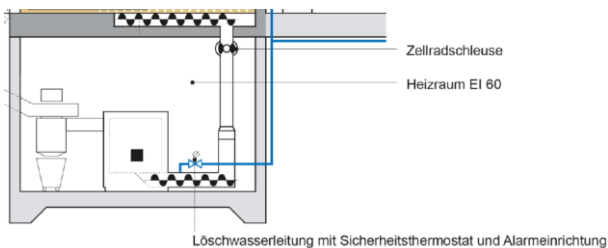
Bild 6.38 Rückbrandsicherung, Fallschacht, Zellradschleuse (Quelle: VKF 104-15 Spänefeuerungen [70]).
