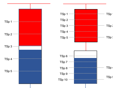
Bild 7.12 Empfohlene Anordnung von 5 Temperaturfühlern bei einem Speicher (links) und von zehn beziehungsweise fünf Temperaturfühlern bei zwei Speichern in Serie (rechts).
