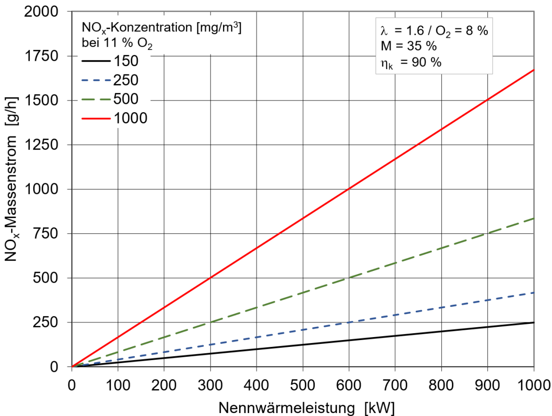
Bild 20.6 NO x -Massenstrom in g/h in Funktion der Nennwärmeleistung in kW und verschiedener NO x -Konzentrationen.
