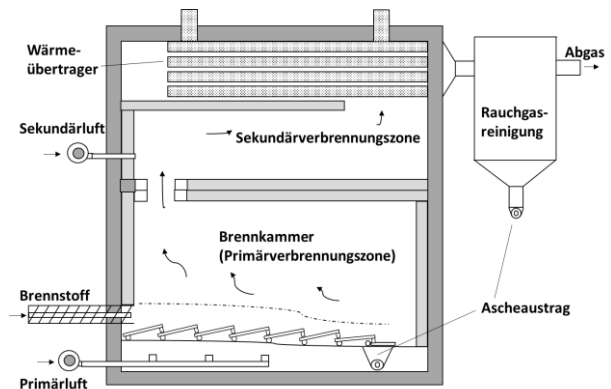
Bild 5.6 Funktionsprinzip einer Vorschub-Rostfeuerung.
