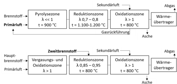
Bild 5.13 Prinzip der Luftstufung (oben) und Brennstoffstufung (unten) zur Reduktion von NO x .
