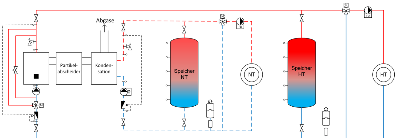
Bild 13.20 Prinzipschema Einbindung Abgaskondensation in ein Niedertemperaturnetz.
