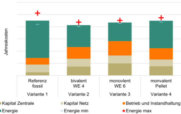
Bild 10.3 Jahreskosten mit Sensitivitätsvergleich «Energiepreise».
