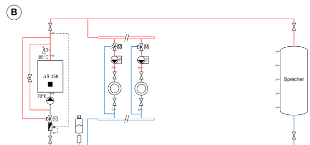
Bild 7.16 Hydraulische Einbindung Wärmespeicher – Schaltung B.
