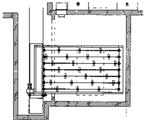
Bild 6.22 Siloaustragung durch Kratzboden [68].
