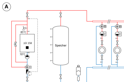
Bild 7.15 Hydraulische Einbindung Wärmespeicher – Schaltung A.
