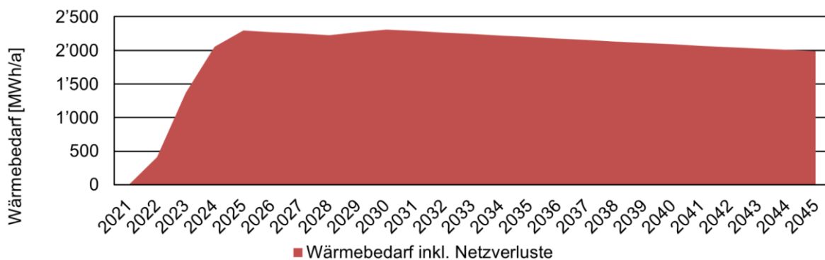
Bild 10.7 Entwicklung des Wärmeverkaufes. Aufgrund von Sanierungen und Effizienzmassnahmen der Wärmekundschaft, nimmt der Wärmeverkauf über die Jahre ab, wenn keine neuen Liegenschaften angeschlossen werden.
