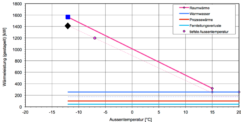
Bild 13.4 Bestimmung der erforderlichen Gesamtkesselleistung bei einer bivalenten oder monovalenten Holzkesseanlage mit Hilfe der Lastkennlinie).
