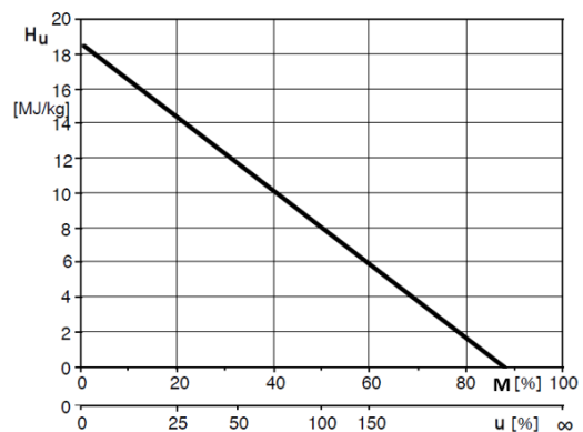
Bild 4.2 Heizwert von Holz in Funktion des Wassergehalts M und der Holzfeuchte u.
