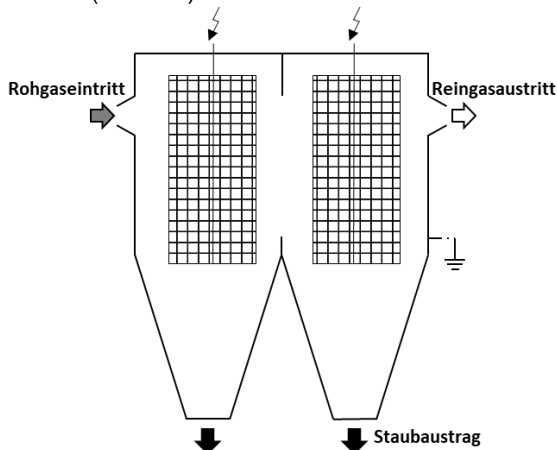
Bild 5.18 Schema eines Elektroabscheiders.
