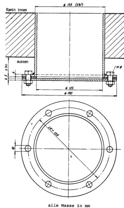
Bild 13.33 Einbaumasse EMPA-Normstutzen [68].
