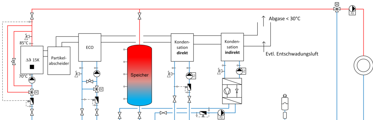
Bild 13.25 Prinzipschema Einbindung Wärmepumpe in die Abgaskondensation.
