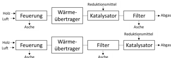
Bild 5.21 Selective Catalytic Reduction (SCR) high-dust-Verfahren (oben) und low-dust-Verfahren (unten).
