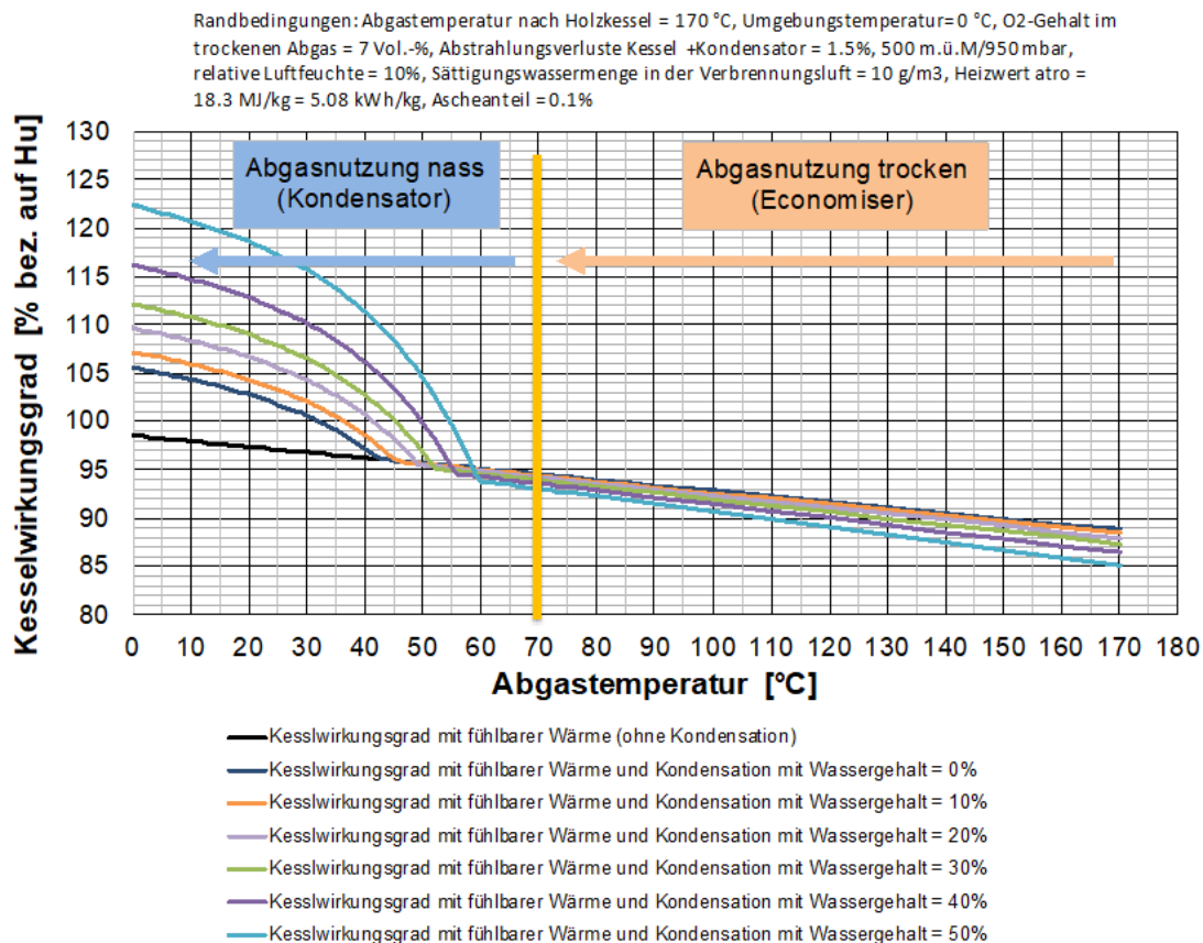
Bild 13.15 Kesselwirkungsgrad in Funktion der Abgastemperatur und des Wassergehalts. Trockene Abgasnutzung mit Economiser, nasse Abgasnutzung mit Abgaskondensation (Quelle Verenum AG).
