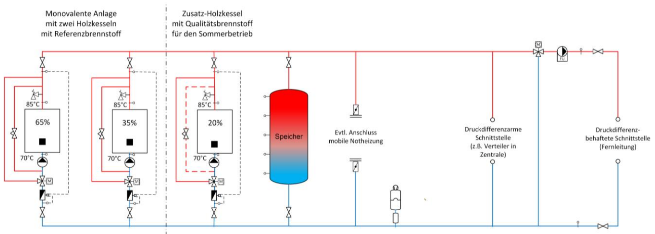
Bild 13.13 Prinzipschema einer monovalenten Anlage mit zwei Holzkesseleln sowie mit einem Zusatz-Holzessel mit Qualitätsbrennstoff für den Sommerbetrieb.
