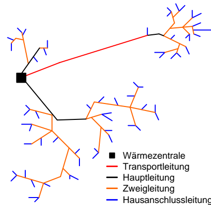
Bild 8.1 Netzaufbau und Leitungstypen [19].
