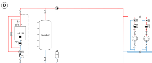
Bild 7.18 Hydraulische Einbindung Wärmespeicher – Schaltung D.
