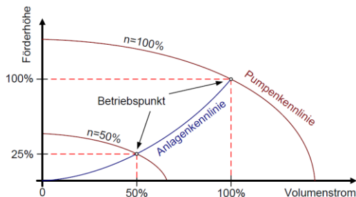
Bild 7.7 Pumpen- und Anlagenkennlinie für zwei verschiedenen Drehzahlen [19].
