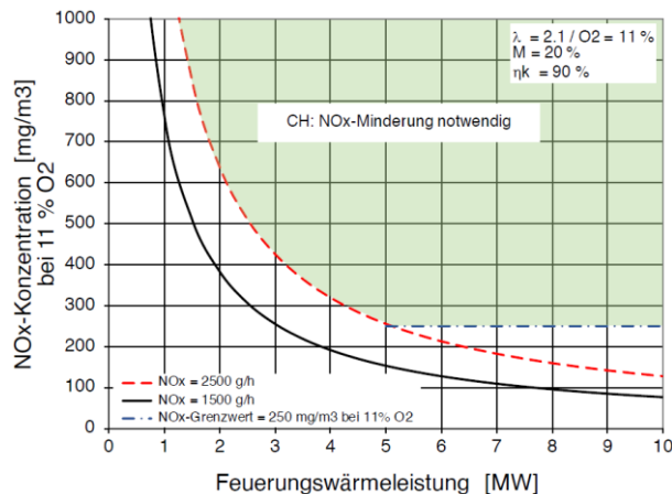
Bild 13.28 NO x -Konzentration in Funktion der Feuerungswärmeleistung als Kriterium für NO x -Minderungsmassnahmen.
