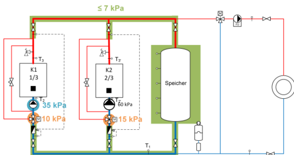
Bild 7.2 Kesselkreise mit konstantem Durchfluss bei Mehrkesselanlagen. Kessel 1 wird beim Parallelbetrieb der beiden Kessel bei Kesselnennleistung beeinflusst, respektive wesentlich reduziert.
