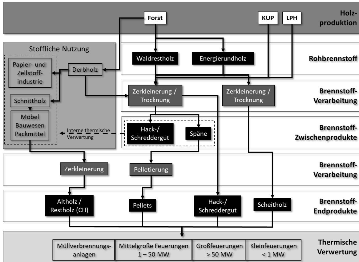
Bild 4.3 Stoffflussdiagramm Energieholz.
