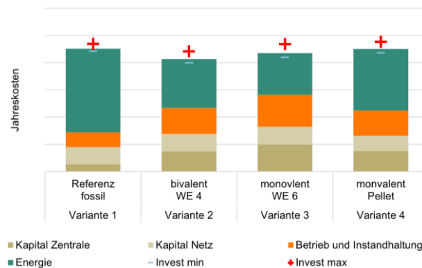
Bild 10.4 Jahreskosten mit Sensitivitätsvergleich «Investitionskosten».
