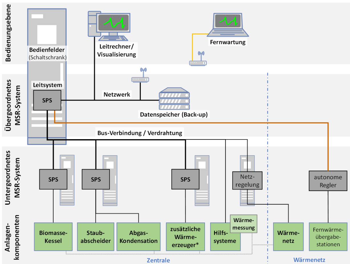
Bild 5.23 Funktionsbezogene Unterteilung eines Prozessleitsystems in Bedienungsebene, übergeordnetes MSR-System und untergeordnete MSR-Systeme (Beispiel für ein Holzheizwerk mit Wärmenetz).
