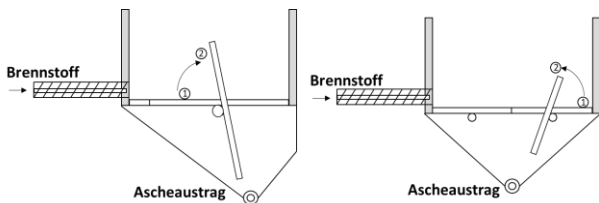
Bild 5.5 Funktionsprinzip der Brennstoffbelegung und Entaschung beim Kipprost (links) oder Stufenbrecherrost (rechts); (1) geschlossene Position, (2) offene Position.
