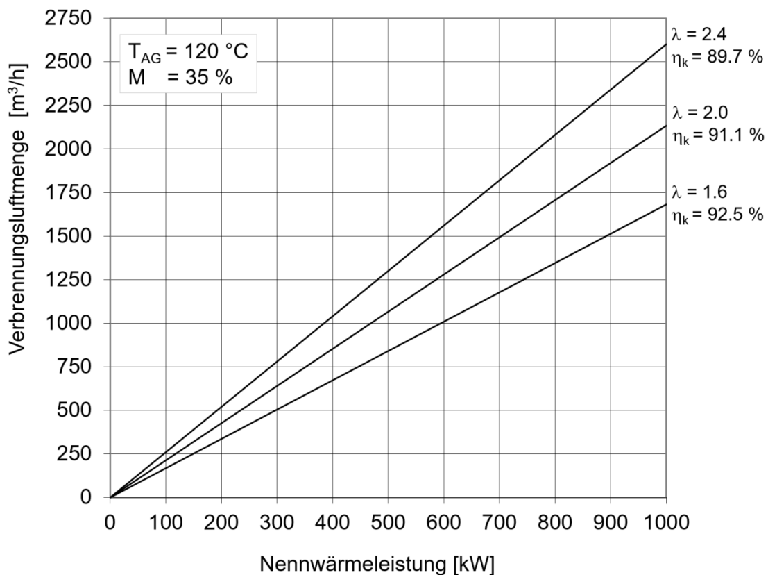
Bild 20.3 Verbrennungsluftmenge in Funktion von Nennwärmeleistung und Luftüberschusszahl
