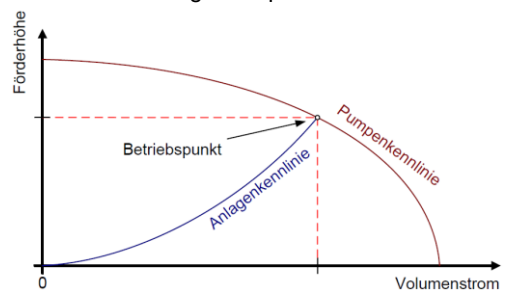
Bild 7.6 Pumpen- und Anlagenkennlinie [19].
