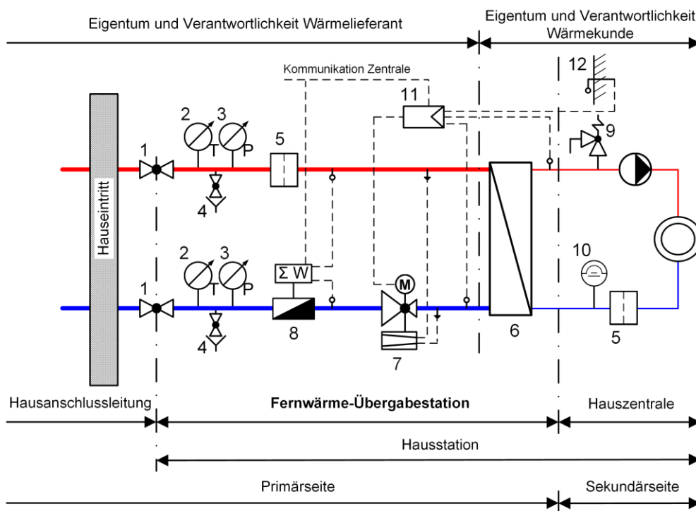
Bild 8.2 Minimalanforderung Fernwärme-Übergabestation [76].
