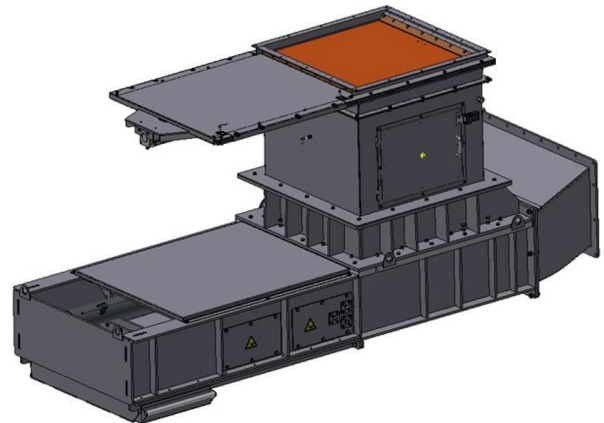
Bild 6.36 Beschickung mit hydraulischem Einschieber (Quelle: Schmid energy solutions).
