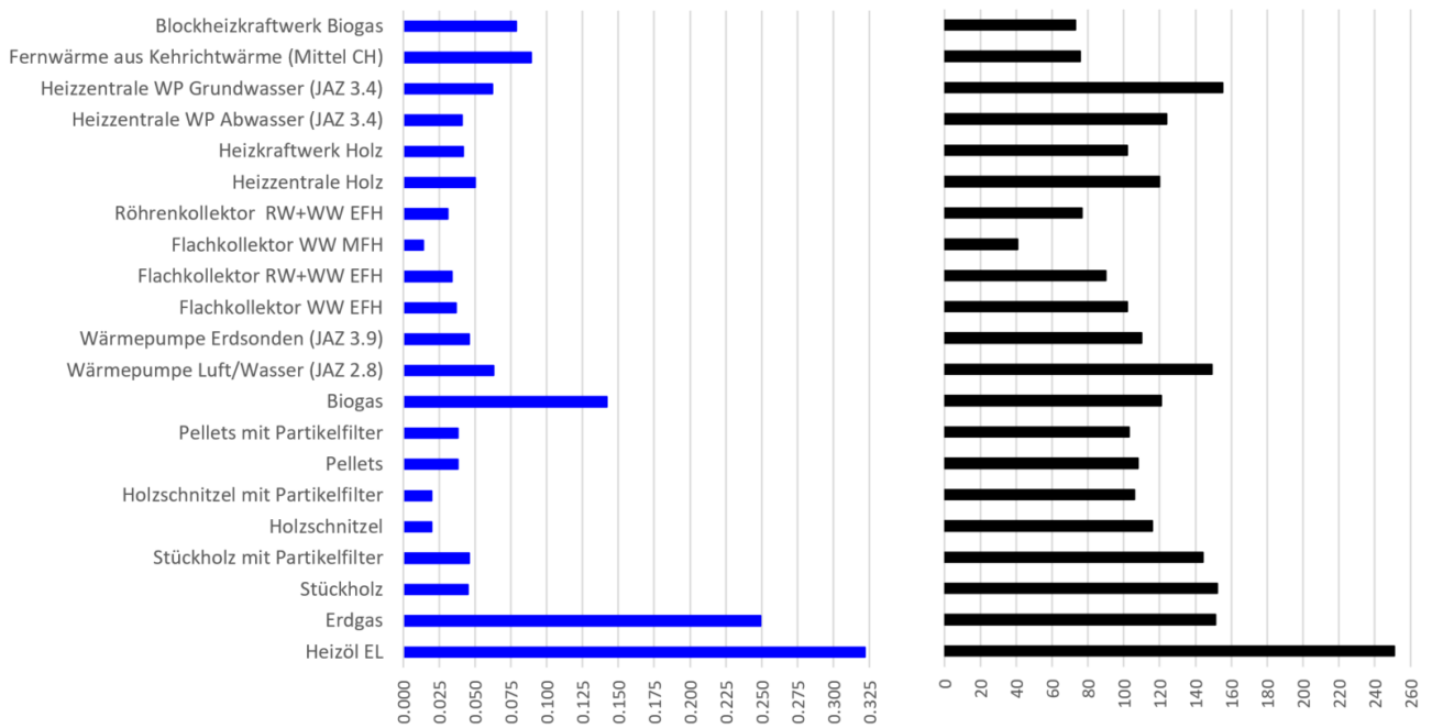
Bild 13.3 Links (blau): Treibhausgasemissionen in [kg\ CO_2\text{-eq}/kWh_{Nutzwärme}] Rechts (schwarz): Umweltbelastungspunkte [UBP/kWh_{Nutzwärme}] nach Tabelle 13.2
