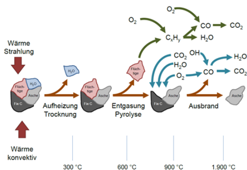
Bild 5.2 Vereinfachtes Verbrennungsprozessschema.
