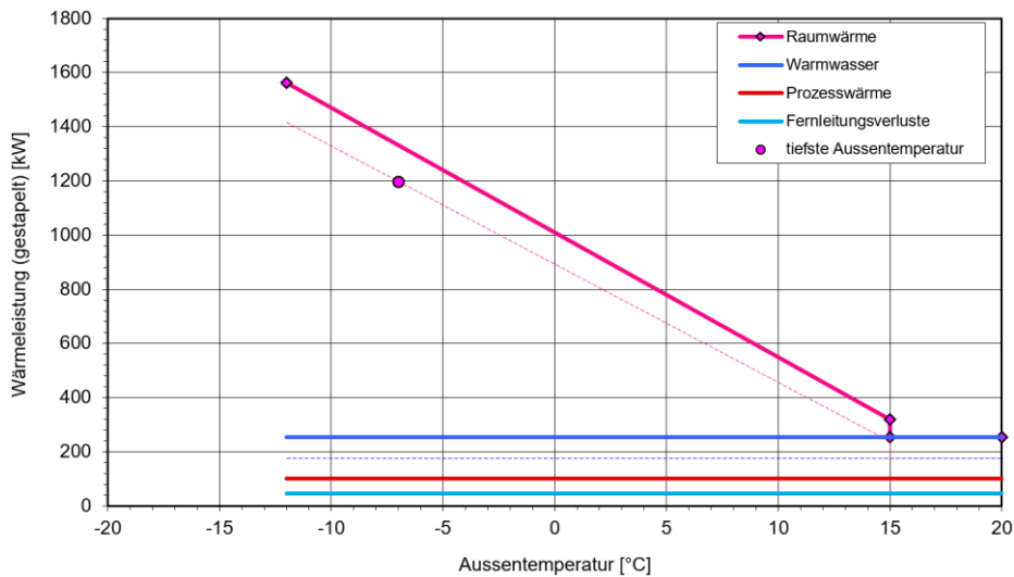
Bild 11.1 Ausgezogen die Lastkennlinie der Gesamtanlage, gestrichelt die gewichtete Lastkennlinie zur Berechnung der Jahresdauerlinie der benötigten Wärmeleistung.
