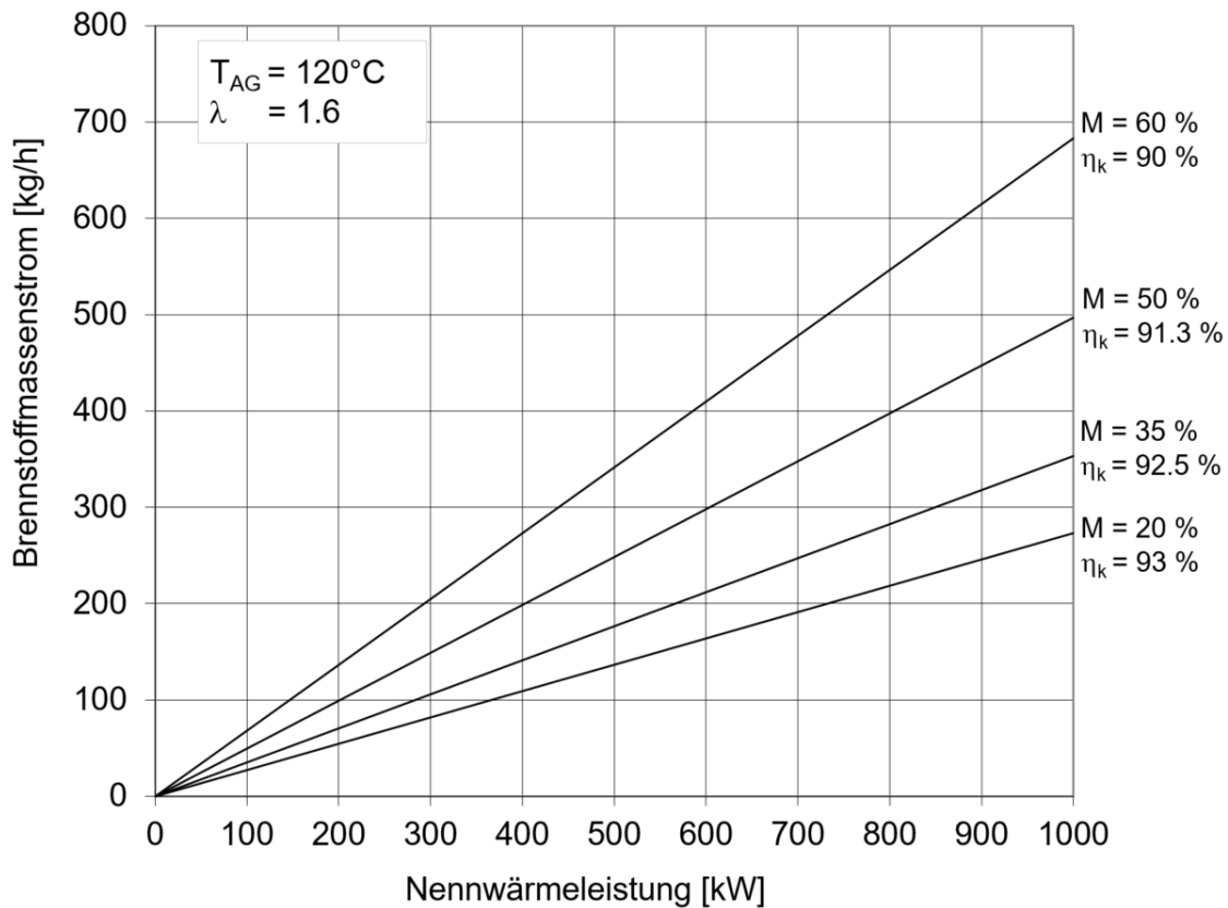
Bild 20.2 Brennstoffmassenstrom in Funktion der Nennwärmeleistung
