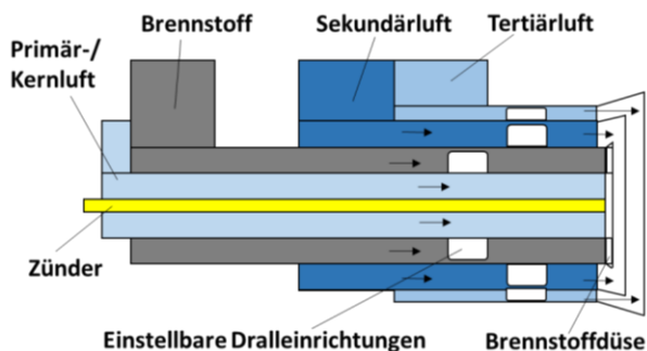
Bild 5.9 Schnitt durch einen Drallbrenner.
