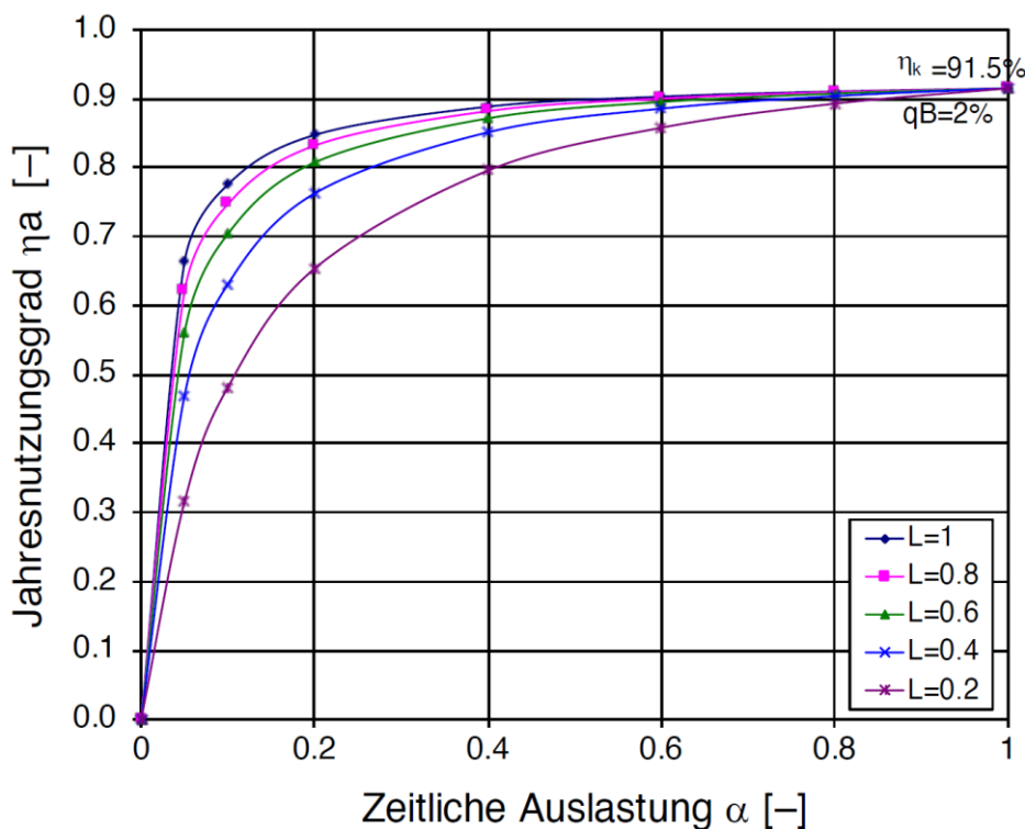
Bild 20.9 Jahresnutzungsgrad eines Holzkessels in Abhängigkeit seiner zeitlichen Auslastung [147] mit \eta_k : Kesselwirkungsgrad; q_B : Bereitschaftsverluste; L : Mittlere Laststufe.
