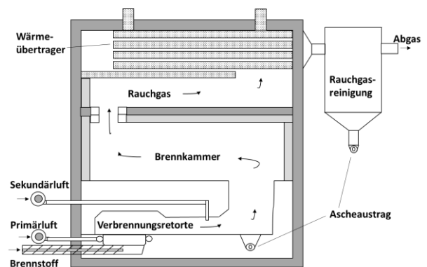
Bild 5.4 Funktionsprinzip einer Unterschubfeuerung.
