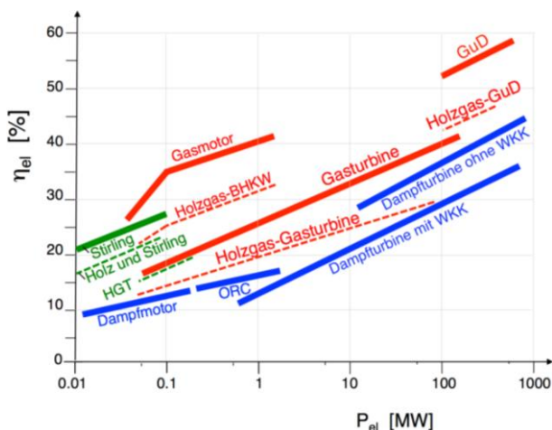
Bild 13.14 Elektrische Netto-Wirkungsgrade verschiedener Technologien zur Stromerzeugung in Funktion der elektrischen Leistung [19]. GuD = Gas- und Dampf-Kombikraftwerk, HGT = Heissgasturbine (mit Holzverbrennung).
