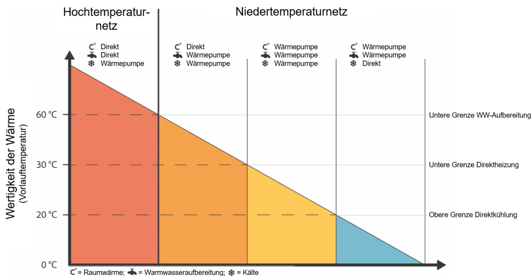
Bild 12.5 Einteilung thermischer Netze in Funktion der Vorlauftemperatur (nach [126] mit Ergänzungen).
