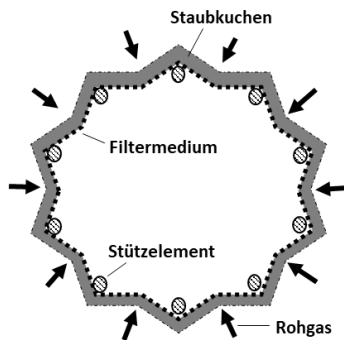
Bild 5.17 Schnitt durch einen Filterschlauch.
