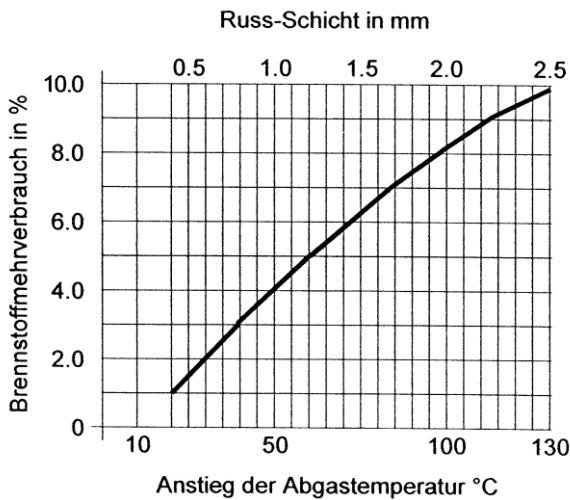
Bild 17.2 Zusammenhang von Russ-Schicht auf den Wärmetauschern, Brennstoffmehrerbrauch und Anstieg der Abgastemperatur im Kessel.
