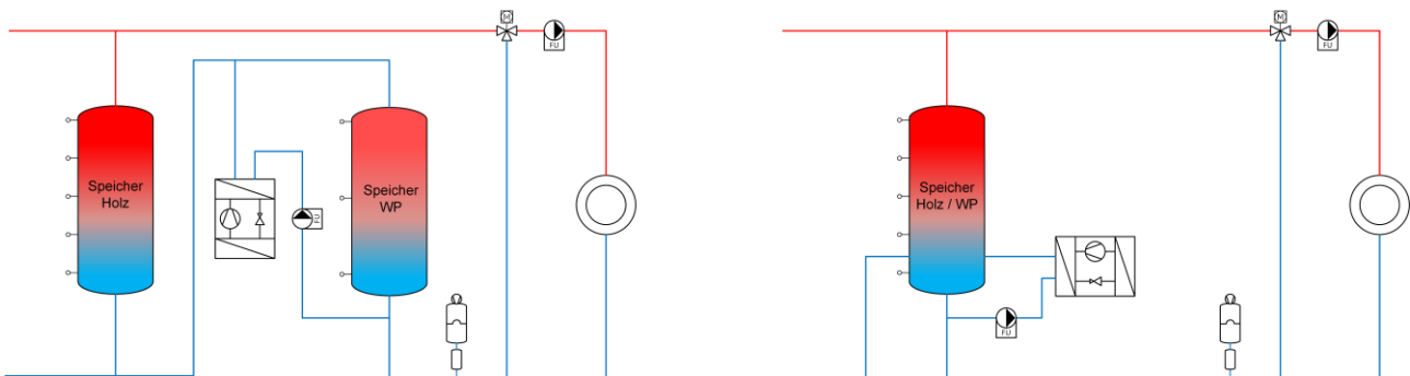
Bild 13.21 Prinzipschema zur Einbindung von Wärmepumpen.
