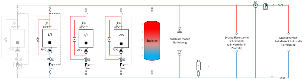
Bild 13.9 Prinzipschema einer Anlage mit mehreren Holzkesseln und mit Speicher (WE6+).
