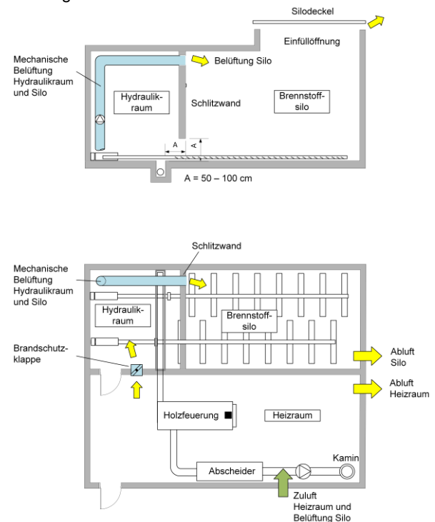
Bild 13.30 Kombinierte Heizraum- und Silobelüftung.
