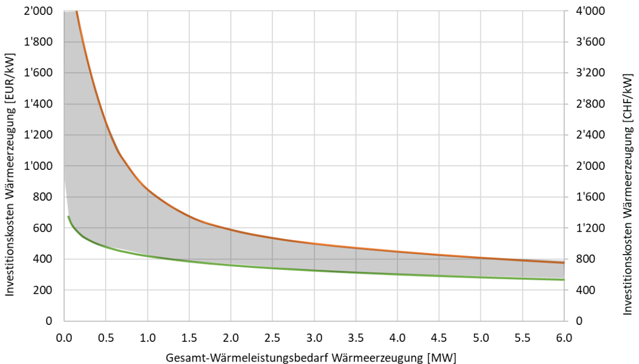
Bild 10.8 Spezifische Investitionskosten Wärmeerzeugung – Auswertung realisierter Anlagen aus AT und CH im Zeitraum 2009 - 2018.
