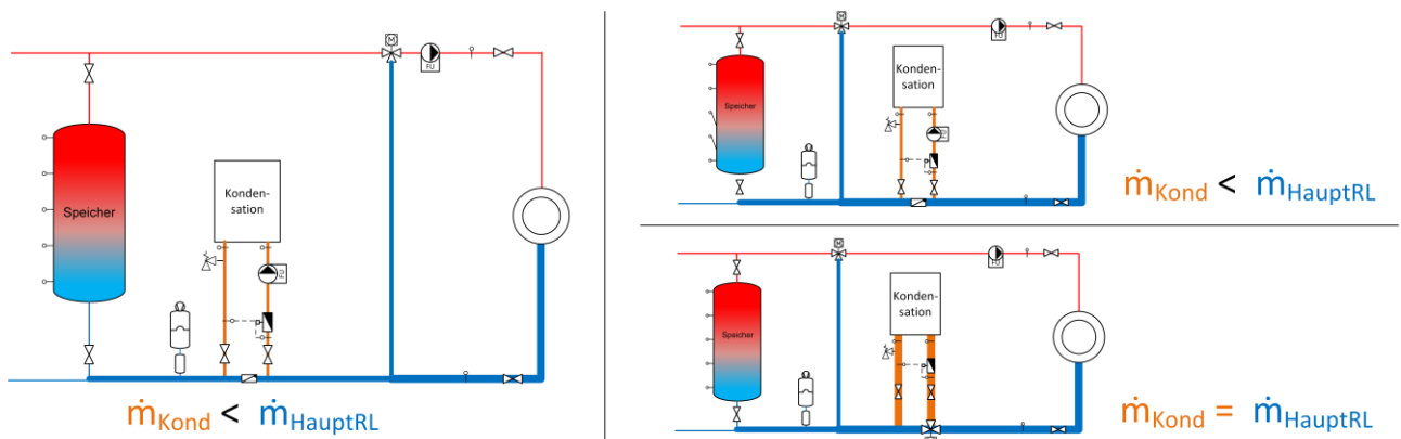
Bild 13.19 Prinzipschema mit Einbindung der Abgaskondensation in den Haupt-Rücklauf vor dem Speicher.
