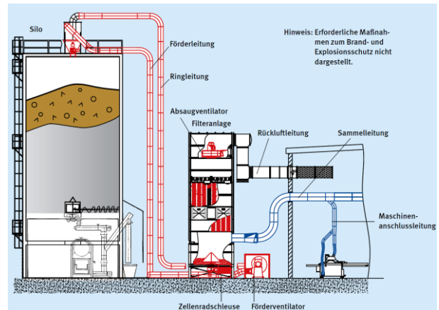
Bild 6.19 Silobefüllung mit betriebseigener Späneabsauganlage (Quelle: BGI 739-2 [69]).
