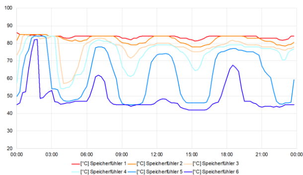
Bild 7.13 Zeitverlauf der Temperaturen im Wärmespeicher beim Laden und Entladen.
