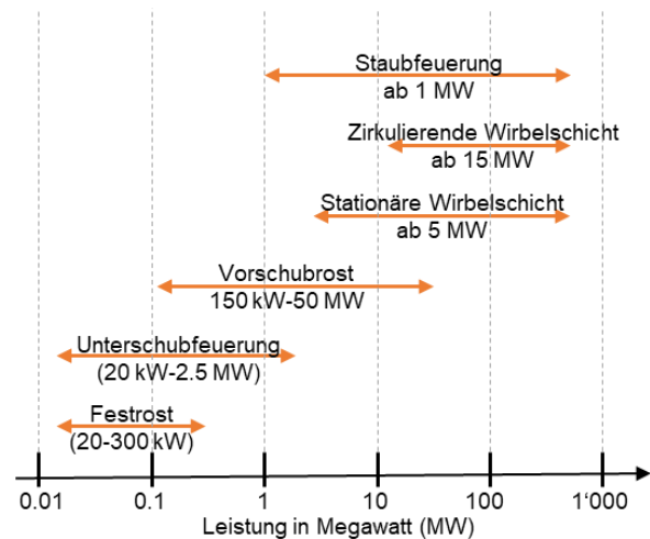
Bild 5.1 Einsatzgebiete der wichtigsten Bauarten von Holzfeuerungen.
