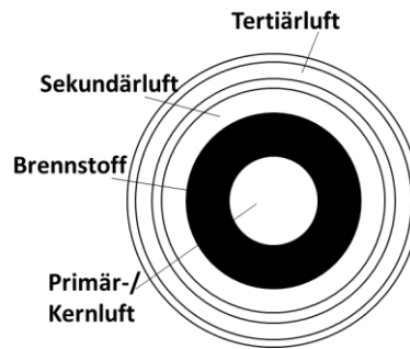
Bild 5.10 Prinzip der Luftstufung innerhalb der Flamme eines Drallbrenners (Blick von vorne auf Luft- und Brennstoffdüsen).
