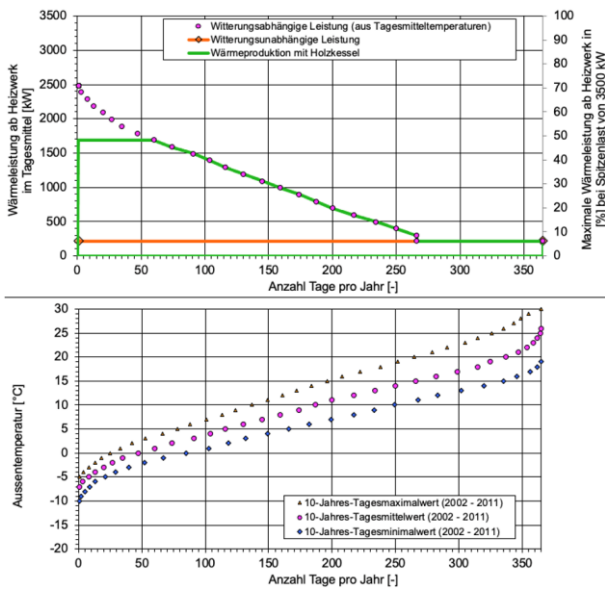
Bild 13.11 Beispielhafte Darstellung der Jahresdauerlinie eines bivalenten Holzheizwerkes. Oben: Jahresdauerlinie der Wärmeleistung im Tagesmittel; Unten: Jahresdauerlinie der Aussentemperatur im Tagesmittel.
