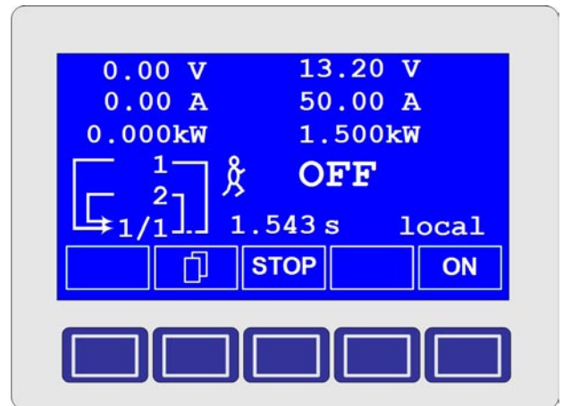
Es wird die abgearbeitete Zeit seit dem Start des Funktionsablaufs angezeigt. Nach einem Stopp wird die Zeit angehalten. Über die STEP , RUN oder GO Taste wird der Funktionsablauf fortgeführt. Die Zeit läuft danach weiter.
