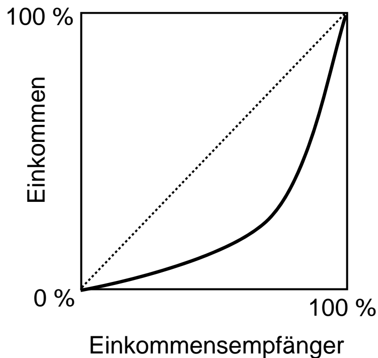
Lorenzkurve vor Besteuerung
