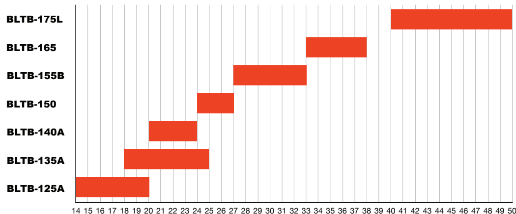
Baggerdienstgewicht/ Applicable Excavator Weight in t
