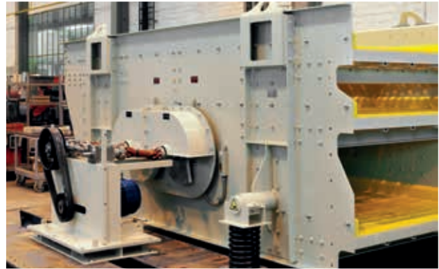
Ellipsenschwingsiebmaschine Typ E, mechanisch einstellbar
