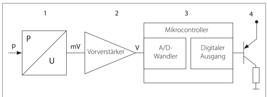
Blockschaltbild
