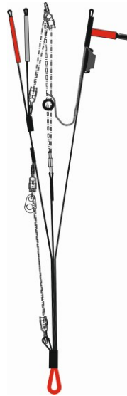
Fig. 3 STELLAR RS riser
