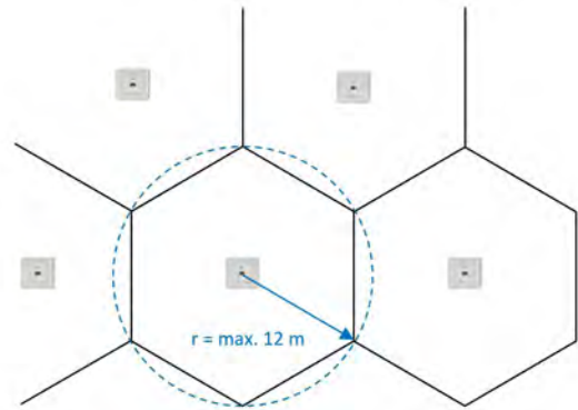
Verteilung von Anschlüssen für WLAN-Access-Points nach DIN EN 50173-6:2018-10. Statt Waben können auch andere Formen wie Kreise, Quadrate oder ähnliche für die Planung verwendet werden.
