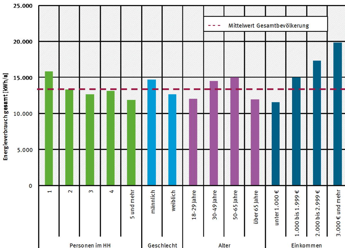
Abbildung 19: Energieverbrauch gesamt
