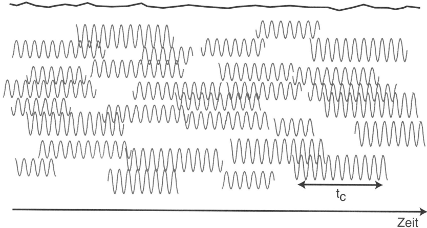
Bild 4.32: Bei monochromatischem Licht aus klassischen Lichtquellen findet man keine einfache Sinuswelle, sondern einen Zug von Wellenstücken, die eine mittlere Dauer von t_c besitzen.
