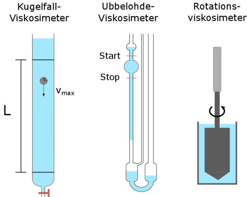
Abbildung 1: Die Abbildung zeigt den schematischen Aufbau des Kugelfall-Viskosimeters, des Ubbelohde-Viskosimeters und des Rotationsviskosimeters.
