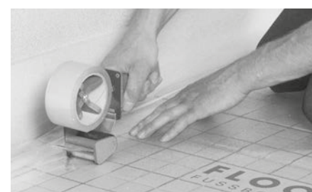
Abb. 2 Folienschürze abkleben
