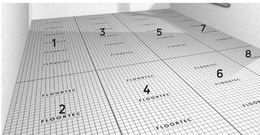
Abb. 2: Kreuzfugenverlegung
