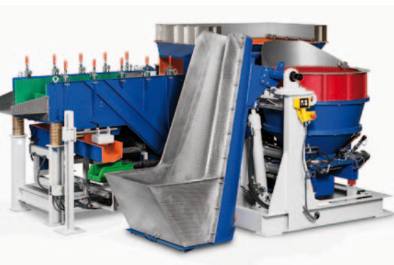
Fliehkraftanlage Baureihe TT/ A 2-C
