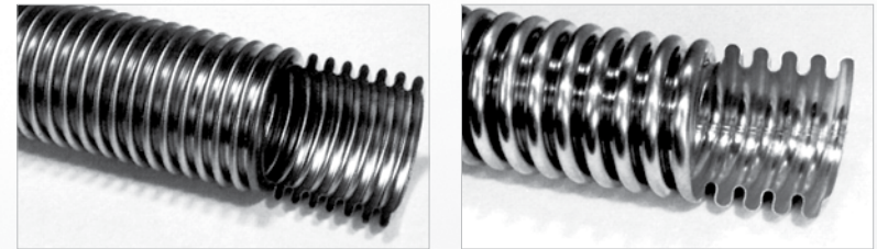
Bild 2.2.1 Ringwellschlauch (links) und Wendelwellschlauch (rechts)
