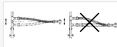
Bild 4.7.10 Laterale Dehnungsaufnahme mit richtig vorgespannter (links) und ungünstig eingebauter Schlauchleitung (rechts)
