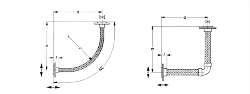
Bild 4.6.1 Metallschläuche zur Schwingungsaufnahme: Ringwellschlauchleitung im 90^\circ -Bogen (links), Ringwellschlauchleitungen mit 90^\circ -Winkel (rechts)
