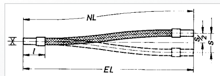
Bild 4.4.1 Laterale Bewegungsaufnahme durch eine Schlauchleitung
