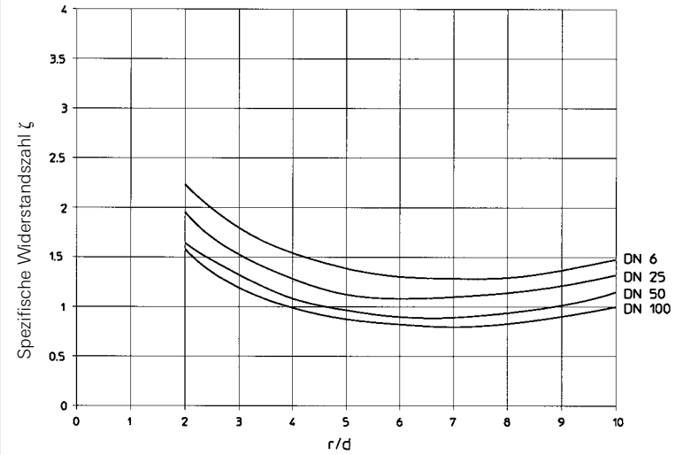
Bild 4.2.6 Spezifische Widerstandszahl \zeta für HYDRA Metallschläuche RS 321
