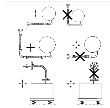
Bild 4.7.12 Lagerrichtiger (linke Teilbilder) und fehlerhafter Einbau (rechte Teilbilder) von Schlauchleitungen zur Schwingungsaufnahme
