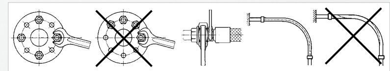
Bild 4.7.5 Torsionsfreie (linke Teilbilder) und fehlerhafte Montage (rechte Teilbilder) der Anschlussflansche
