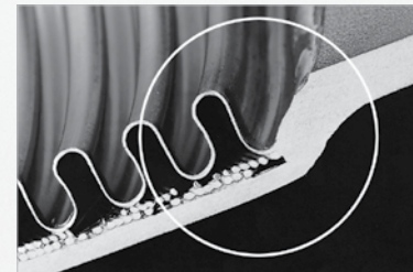
Bild 3.1.5 Spalt- und gratfreie Anbindung eines Metallschlaches
