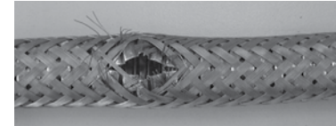
Bild 4.1.1 Bersten des Schlauches unter dem Geflecht
