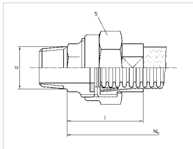
Typ RE58W
