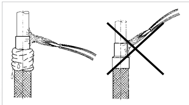
Bild 4.7.6 Korrektes (links) und fehlerhaftes Einlöten (rechts) einer Schlauchleitung
