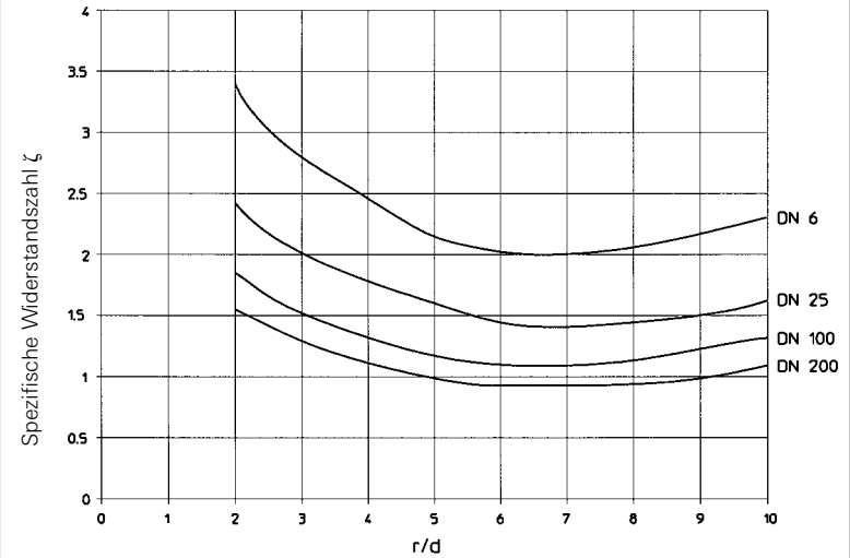
Bild 4.2.10 Spezifische Widerstandszahl \zeta für HYDRA Metallschläuche RS 531/430
