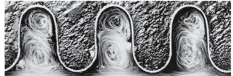
Bild 4.2.2 turbulente Strömung mit ungestörter Kernströmung sowie Primär- und Sekundärwirbeln in den Wellen in einem Ringwellschlauch
