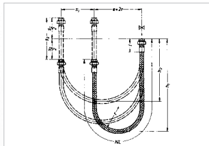
Bild 4.3.4 Horizontale und vertikale Bewegungsaufnahme im vertikalen U-Bogen
