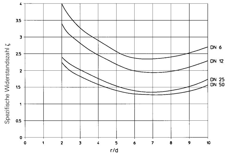
Bild 4.2.8 Spezifische Widerstandszahl \zeta für HYDRA Metallschläuche RS 341
