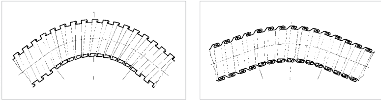
Bild 2.6.2 Bewegung des Wickelschlauhes durch Verschiebung der Windungen relativ zueinander für ein Hakenprofil (links) und ein Agraff-Profil (rechts)
