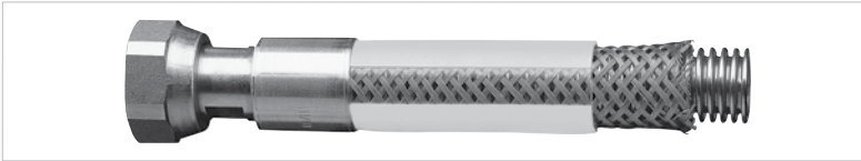
Bild 3.4.6 Dreischichtiger Aufbau der Gasschläuche HYDRAGAS GA 7xx
