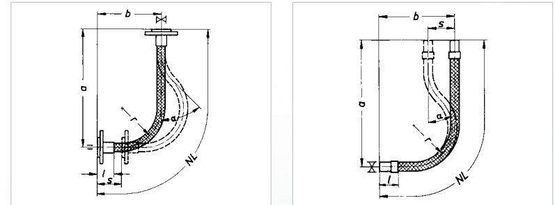
Bild 4.4.2 Einseitige Bewegungsaufnahme durch eine Schlauchleitung im 90°-Bogen
