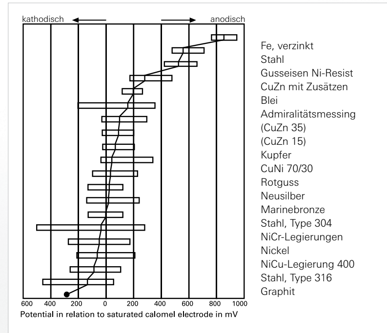
Galvanische Spannungsreihe in Meerwasser Quelle: DECHEMA-Werkstofftabellen.
