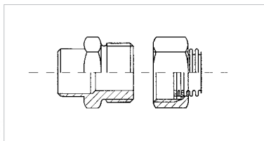
Bild 2 Anschlussverschraubung Einschraubteil mit ISO- Anschweißende oder Stutzen: Typ Präzisionsrohr für Schneidring
