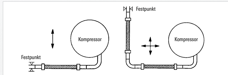
Bild 3.1.13 Montage von HYDRA Schwingungsausgleichern
