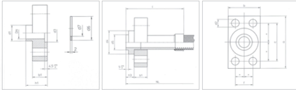
Gegenflansch
