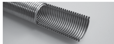
Bild 2.2.3 engewelltes, flexibles Schlauchprofil
