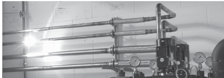
Bild 3.1.12 HYDRA Schwingungsausgleicher im Einsatz
