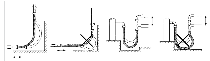
Bild 4.7.3 Kollisionsfreier (linke Teilbilder) fehlerhafter Einbau von Schlauchleitungen (rechte Teilbilder)
