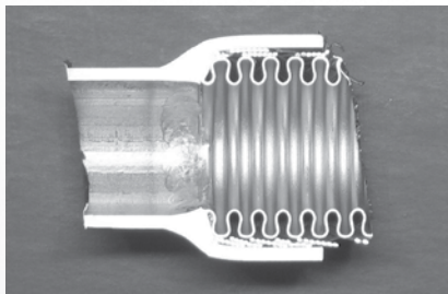
Bild 2.5.3 Schweißanbindung von HYDRA Schlauchleitungen
