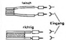
Bild 6. Flachbandkabel dürfen nur kurz vor dem Empfänger aufgetrennt werden
