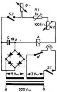
Bild 1. Schaltung des Temperaturüberwachungsgerätes
