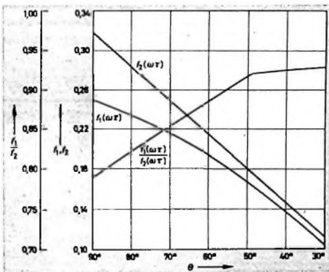
Bild 5. Verlauf der Fourier-Funktionen f_1(\omega\tau) , f_2(\omega\tau) , sowie des Quotienten f_1/f_2 im Bereich der Winkel 90^\circ bis 30^\circ . Man erkennt, daß der Wirkungsgrad unterhalb von 50^\circ annähernd konstant bleibt
