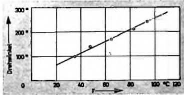
Bild 4. Eichkurve des Überwachungsgerätes
