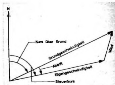
Bild 5. Winddreieck
