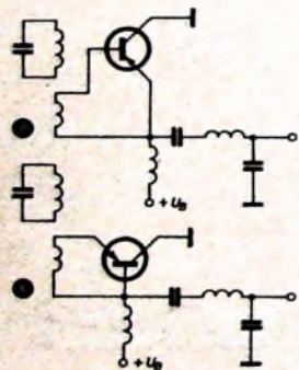
Bild 7. Emitterschaltung (a) und Basischaltung (b) mit geerdetem Collector und Tiefpaßfilter nach Bild 6. Die Spulen am Ein- und Ausgang sind gut zu entkoppeln
