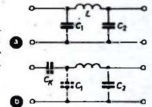
Bild 6. Normales (a) und modifiziertes (b) Tiefpaßfilter, bei dem C_1 als Schaltkapazität aufgelöst ist und mit 2 pF in Rechnung gesetzt wird. Besonders bei der Anpassung sehr niederohmiger Last- und Ausgangswiderstände bietet diese Anordnung Vorteile
