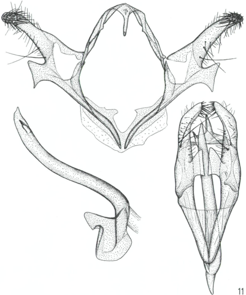
Abb. 11. Calycothra arabicella n. sp., ♂-Genital. Rechts von ventral, Paratypus, GU. Mus. Vind. 3617 ♂. Links Paratypus, GU-4115-Amsel; oben: Valven und Vinculum-Arme auseinandergeklappt (Hülle des Vinculum zerrissen), Aedoeagus und Fultura inferior entfernt; unten: Aedoeagus mit Fultura inferior.
