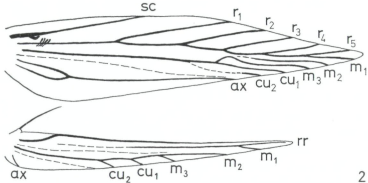
Abb. 2. Geäder von Calyco bathra arabicella n. sp.
