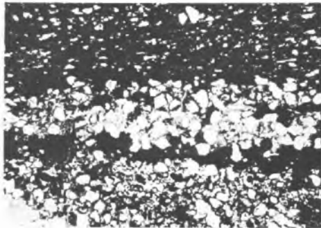
Abb. 4. Quarten-Sandstein mit syngenetischer zyklischer Fällung von kryptokristallinem Hämatit (Roteisenstein), sog. „Gebändertes Eisenerz“. Die hellgrauen, wenig gerundeten Körner sind vorwiegend detritischer Quarz mit etwas Plagioklas und Orthoklas. Die mittelgrauen schummrigen Körner sind vorwiegend Zirkon mit etwas Augit (? tuffogen). Die hell- bis dunkelgraue Grundmasse im mittleren und unteren Bildteil ist chemisch abgesetzter Chlorit. Die schwarze Grundmasse ist Roteisenerz in Form von kryptokristallinem bis feinkörnigem Hämatit. Nicols //, Vergr. ca. 42 ×
