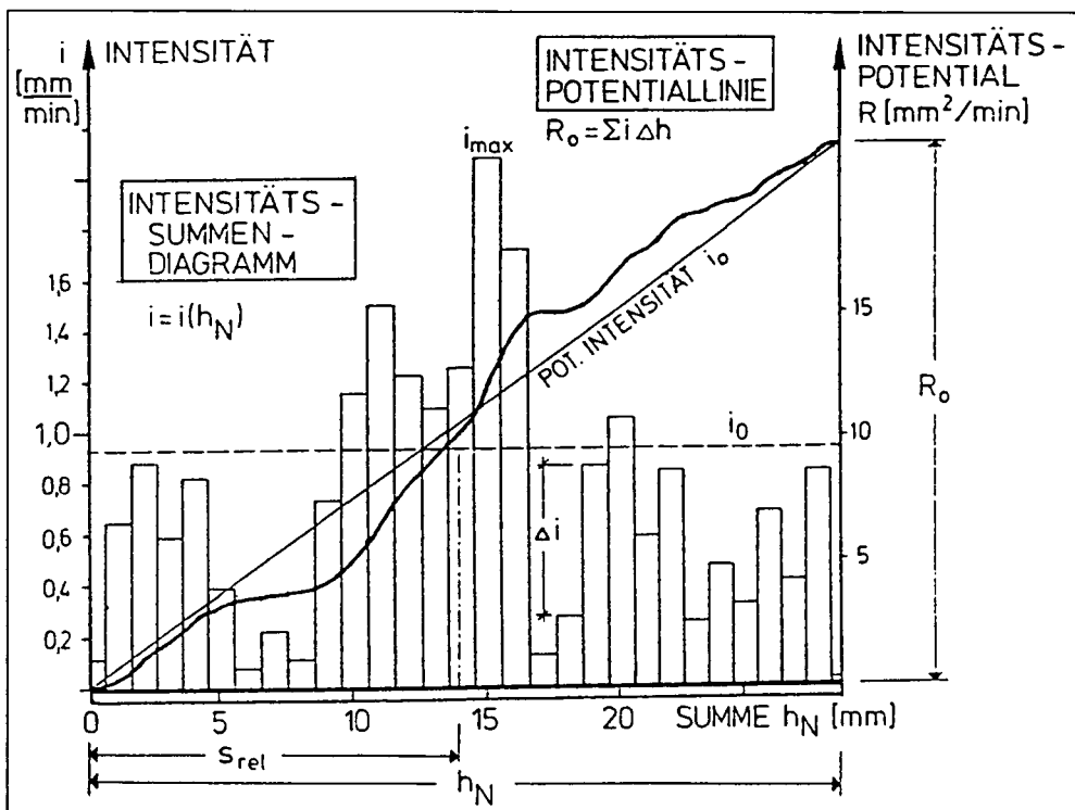
Abb. 3. Intensitätssummendiagramm.
