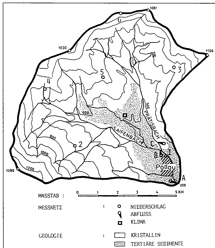
Abb. 1. Hydrologisches Versuchsgebiet Pöllau (Oststeiermark).
