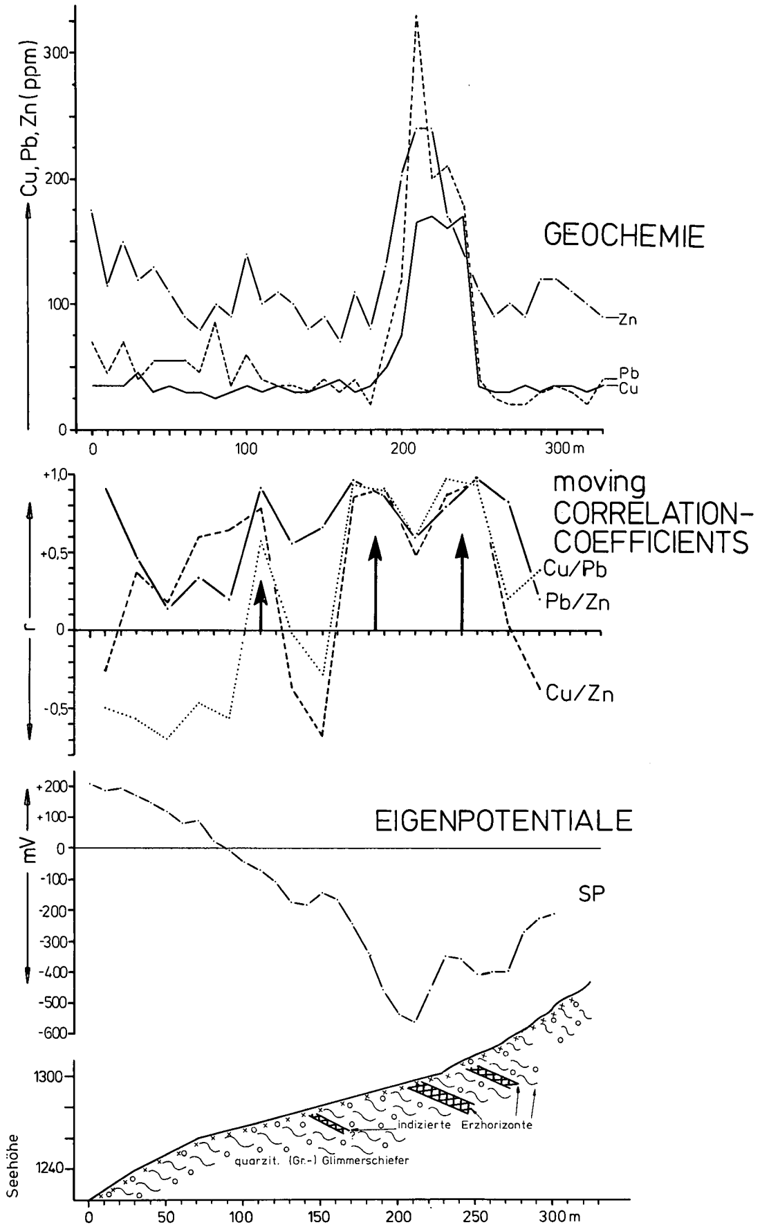
Abb. 3: Vergleich der Ergebnisse von Geochemie, „gleitende Korrelationskoeffizienten“ und SP-Messungen entlang von Profil 20. Die Ergebnisse zeigen deutlich Abhängigkeiten zwischen den stark positiven Korrelationsverhältnissen der Elemente Pb, Zn und Cu, den Maxima der Metallkurven sowie der SP-Anomalie. Obwohl die Migrationseigenschaften der gewählten Indikatorelemente unterschiedlich sind, kommen durch den Glättungseffekt die Unterschiede in den einzelnen Korrelationskurven nicht so stark zum Ausdruck.
