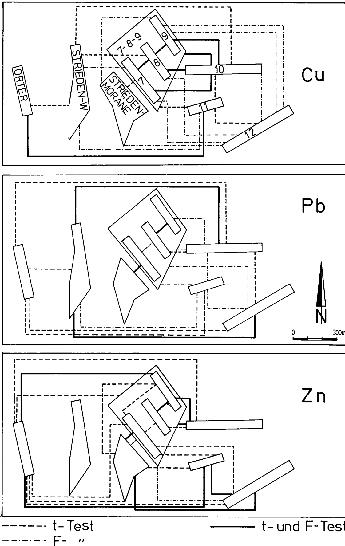
Abb. 2: Student-t- und Snedecor-F-Verteilungsbilder; dargestellt sind die Abhängigkeiten der Parameter \bar{x} und s^2 zwischen Detailbereichen des Suchgebietes. Dabei gilt: t-Test: es bestehen keine signifikanten Unterschiede zwischen den Mittelwerten beider Populationen. F-Test: es bestehen keine signifikanten Unterschiede zwischen den Streuungen beider Populationen. t- und F-Test: beide Populationen gehören einem Kollektiv an.
