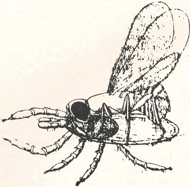
Abb. 1: Ein Weibchen der Schlupfwespe Hunterellus hookeri bei der Eiablage in eine nüchterne Nympe von Ixodes ricinus (nach Brumpt, 1931).
