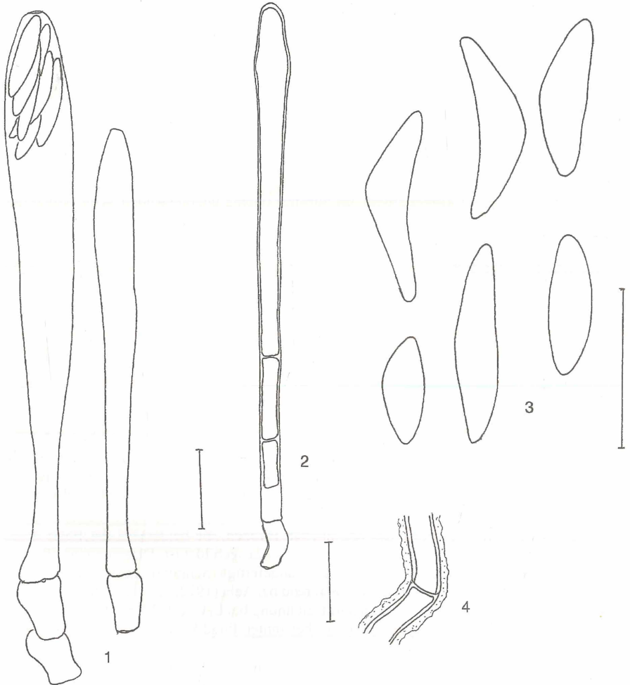
Abb. 5: Mollisia lividofusca (FR.) GILL., Beleg 95/010 AG: 1 - Asci, 2 - Paraphyse, 3 - Sporen, 4 - Teil einer Subikulumhyphe mit Septe. Der Maßstrich entspricht 10 \mu\text{m} .
