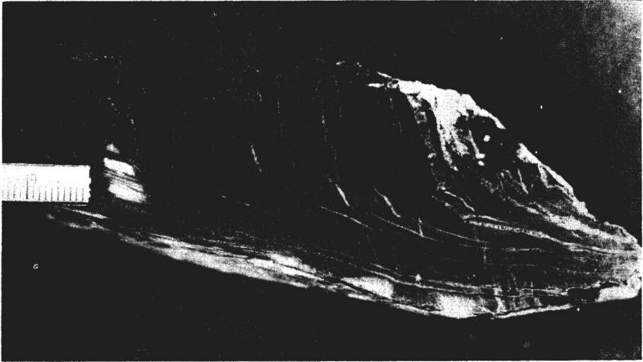
Abb. 7. Materialabhängigkeit des Brechungswinkels (je kompetenter das Material ist, um so größer wird der Brechungswinkel) – Anschliff – Rabisklippen (Bl. Wippra)
