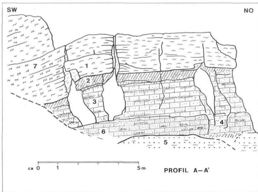
Abb. 4 a: Schematische Skizze des oberen Eingangsbereiches, entsprechend dem Schnitt A-A' in Abb. 2. Die Ziffern 1-7 sind Entnahmestellen von Gesteinsproben: (1) + (7) deutlich geschieferter Biotitgneis (Dach der Höhle). (2) Kalksilikatgestein (Tremolit - Diopsidfels). (3) + (4) + (6) Marmor mit wechselnden Gehalten an Silikaten. (5) Quarzit, der unteren Gneislage angehörend
