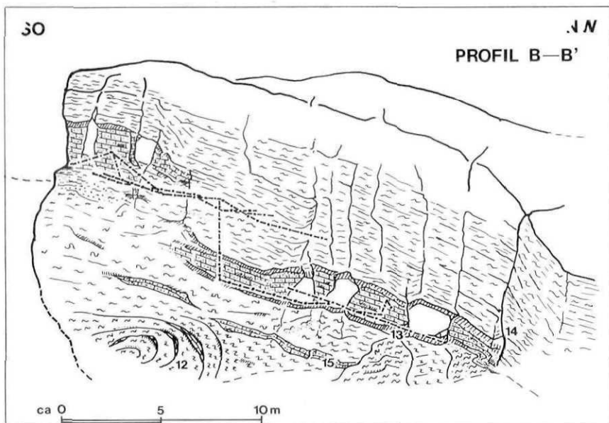
Abb. 4 b: Schematische Skizze des unteren Eingangsbereiches, entsprechend dem Schnitt B – B' in Abb. 2. Die strichpunktiertere Linien stellen die Höhlen-Meßzüge im Seitenriß dar. Die Ziffern 12–15 sind Entnahmestellen von Gesteinsproben: (12) unterlagernder, z. T. stark verfallener Gneis mit Einlagerungen von unterschiedlich mächtigen Quarziten, Marmoren (15) und Kalksilikaten (13). (14) Biotitgneis (Dach der Höhle)
