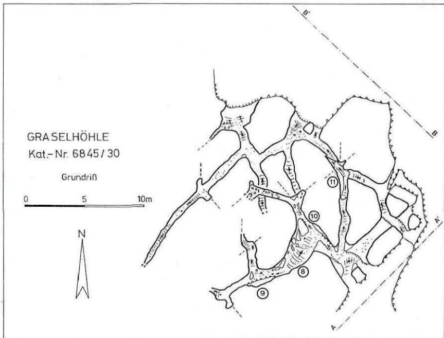
Abb. 2: Grundriß der Graselhöhle (aus Hartmann, H. & W., 1985) mit den eingetragenen Hauptklufrichtungen und Entnahmestellen der in der Höhle genommenen Gesteinsproben (Nr. 8–11). Die Profile A–A' und B–B' sind in den Abb. 4a und 4b dargestellt
