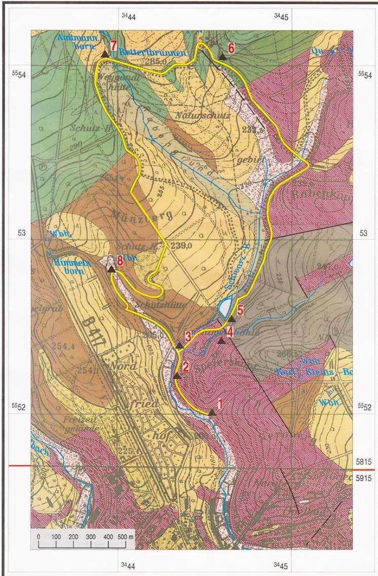
Abbildung 2a: Ausschnitt aus der Geologischen Karte von Hessen 1 : 25 000, Blatt 5815 Wehen (1932) und Blatt 5915 Wiesbaden (1971), für den Bereich Nerotal-Rabengrund mit dem Verlauf des Geopfads und seinen acht Haltepunkten. Die Geologie des Kartenausschnitts wurde entsprechend der neuen Stratigraphie erstellt. Topographische Grundlage: TK25 der Hessischen Verwaltung für Bodenmanagement und Geoinformation, Wiesbaden, Verv.-Nr.: 2001-3-112
