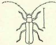
Fig. 61. Stenostola ferrea .
