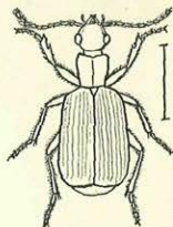
Fig. 19. Brachynus crepitans.
