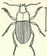
Fig. 18. Poecilus coeruleus.
