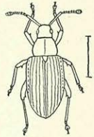
Fig. 62. Phyllobius calcaratus .
