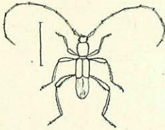
Fig. 59. Caenoptera minor .
