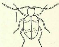
Fig. 55. Ptinus rufi-pes ♀.
