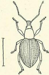
Fig. 63. Otiorrhynchus niger .
