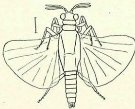
Fig. 69. Xenos vesparum ♂.
