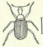
Fig. 65. Apoderus coryli .
