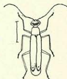
Fig. 51. Malthinus flaveolus .
