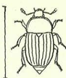
Fig. 29. Silpha obscura.
